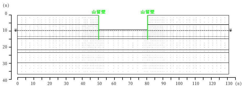
C－C'断面
