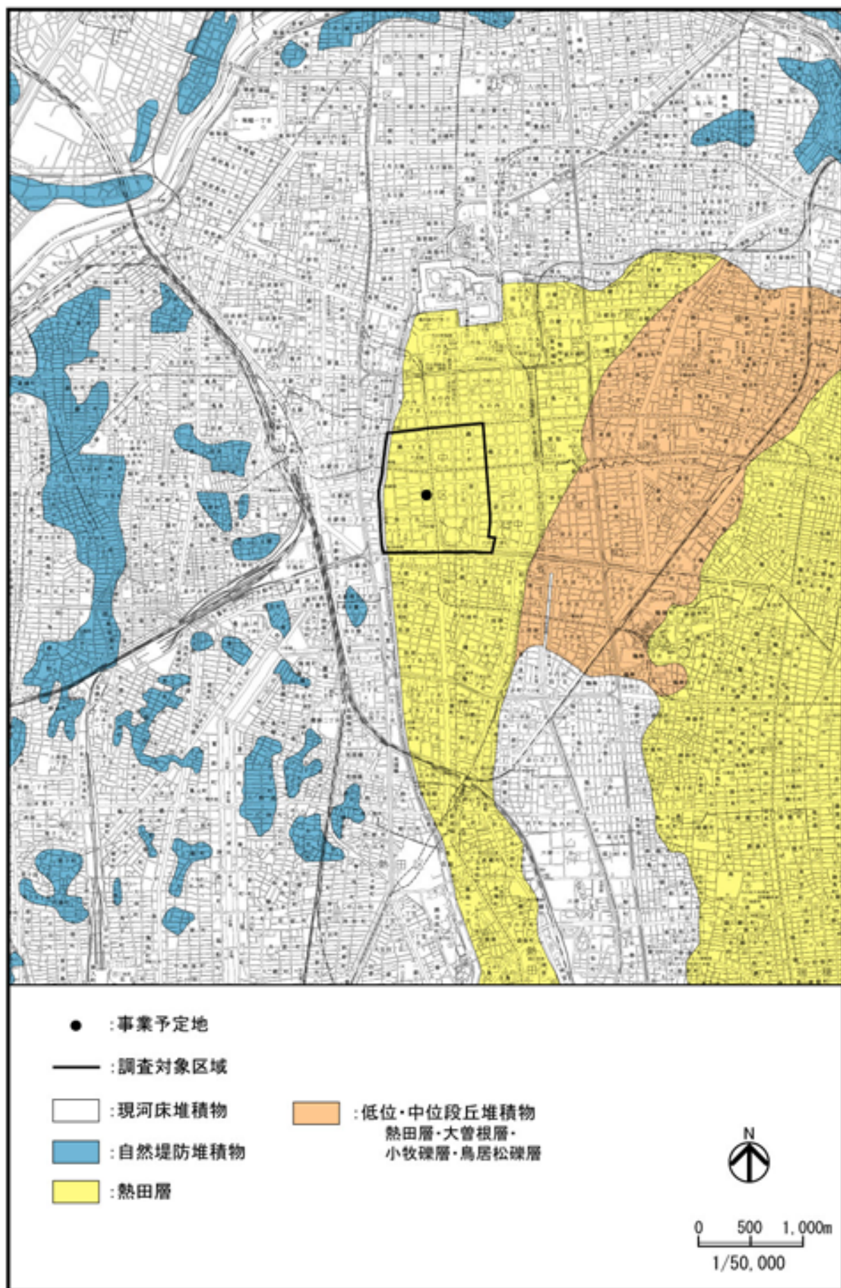
図 1-4-18 表層地質図
