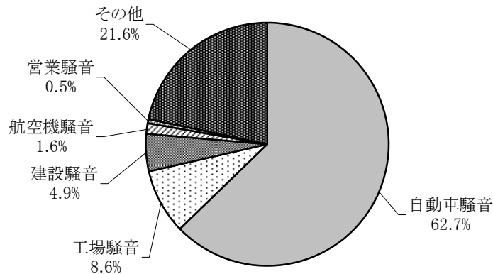
図 1-4-20 環境騒音の主な寄与音源
