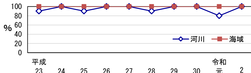
図 1-2 環境基準達成率（河川はBOD、海域はCOD）の10年間の推移
