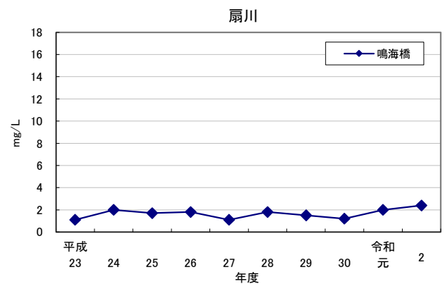
図1-6 (1) 75%水質値 (BOD) の経年推移
