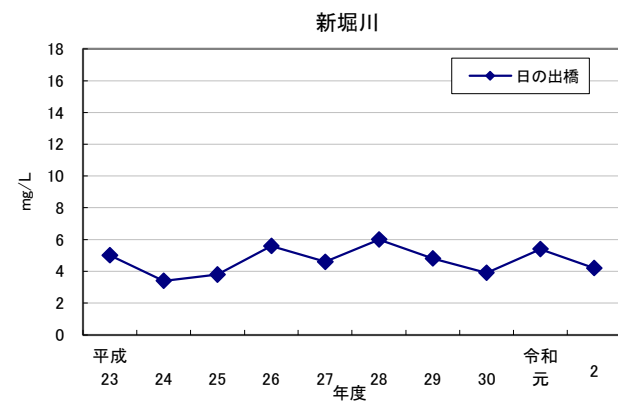
図1-6 (1) 75%水質値 (BOD) の経年推移
