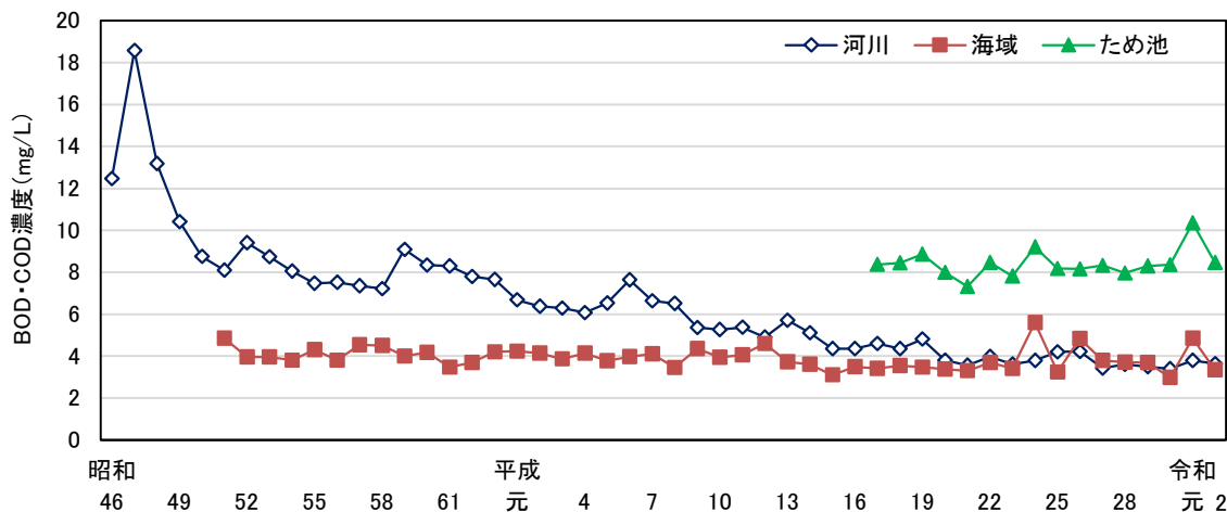
図 1-4 全市年間平均値（河川はBOD、海域・ため池はCOD）の推移
