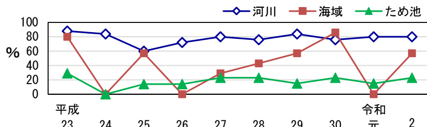
図 1-3 環境目標値達成率（河川はBOD、海域・ため池はCOD）の10年間の推移
