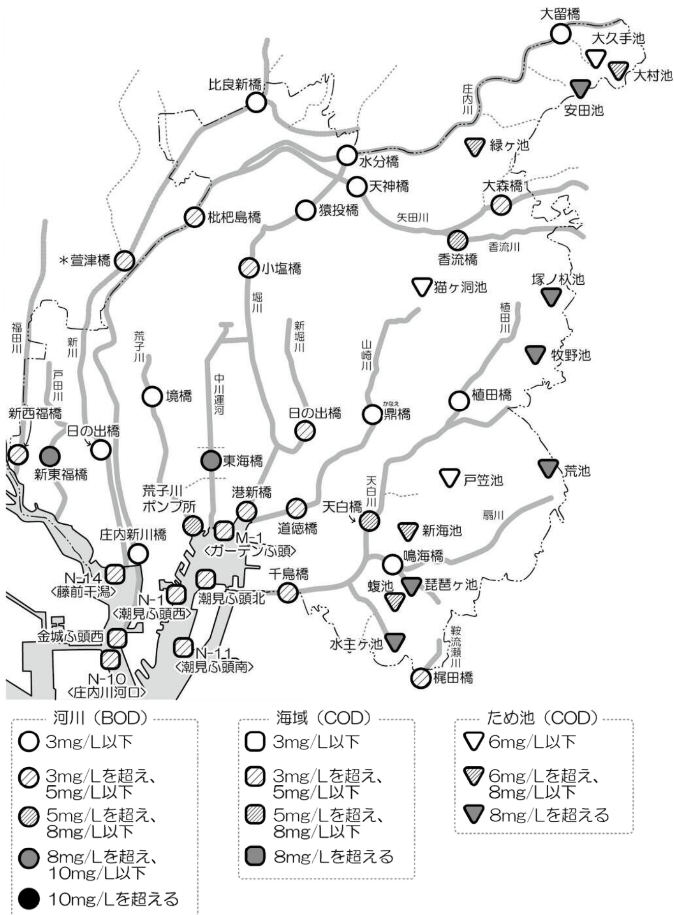
図 1-5 水質の状況 (75%水質値)
