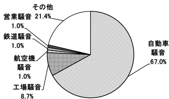
図 3 主な寄与音源
