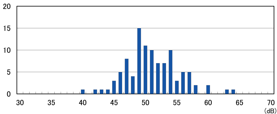
図1 等価騒音レベルの分布状況（昼間）
