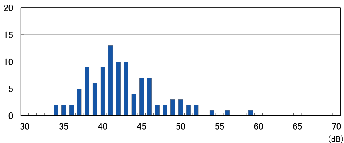
図2 等価騒音レベルの分布状況（夜間）
