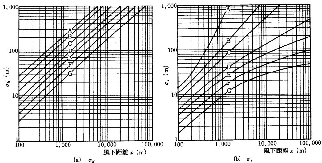
図 3-8-1 Pasquill-Gifford 図
