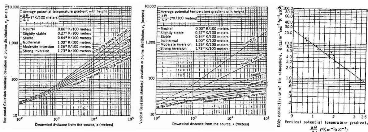
図 3-12-3 カーペンターらによる煙の広がり幅及び渦伝導度
