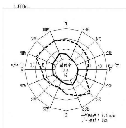
図 3-4-2 高度別風配図 (年間)
