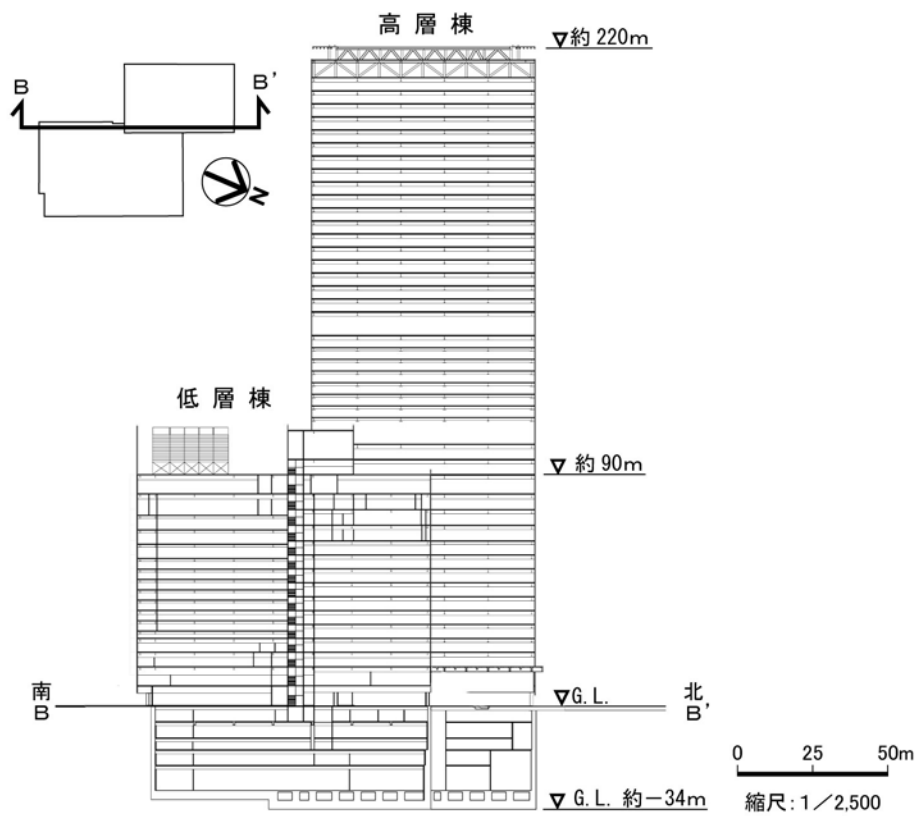
図3-2-4(2) 南北断面図
