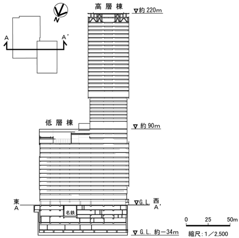
図3-2-4(1) 東西断面図
