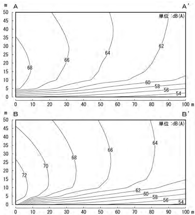
図-2 断面予測結果 (ケース I)
