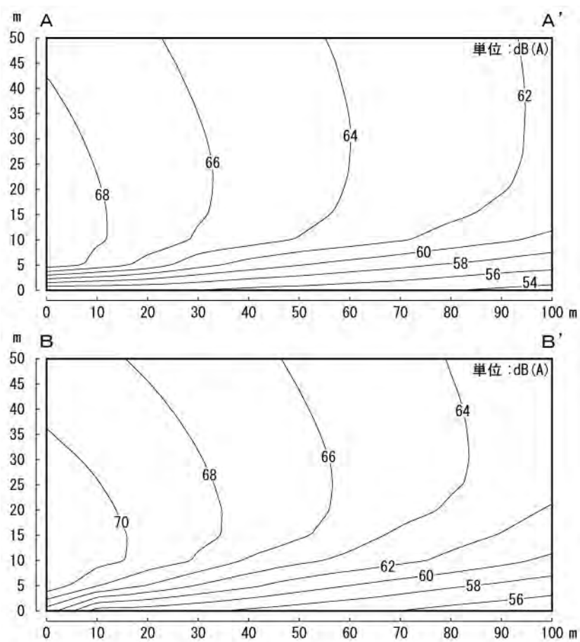
図-3 断面予測結果 (ケース II)
