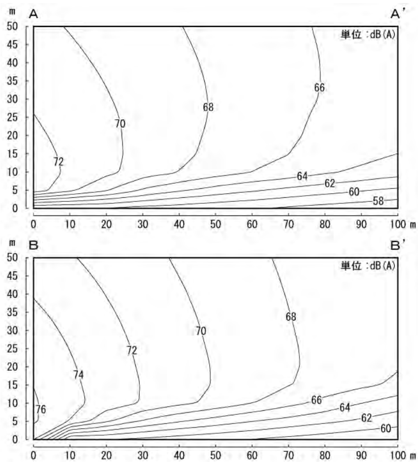
図－4 断面予測結果（ケースⅢ）
