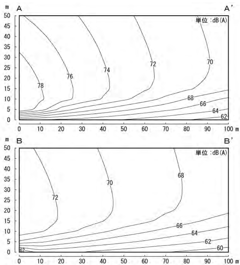
図－5 断面予測結果（ケースⅣ）
