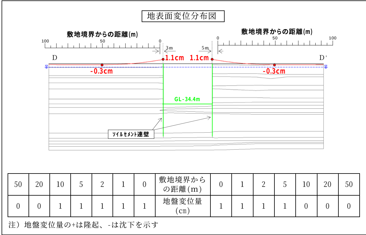
図 2-4-10(4) 掘削工事後の地盤変位 (D-D'断面)
