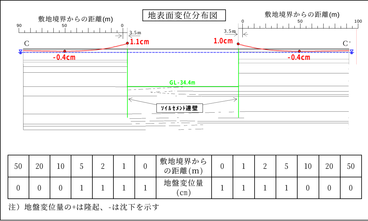
図 2-4-10(3) 掘削工事後の地盤変位 (C-C'断面)
