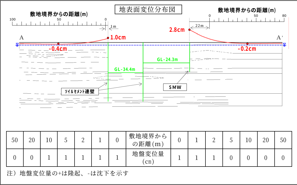
図 2-4-10(1) 掘削工事後の地盤変位 (A-A'断面)
