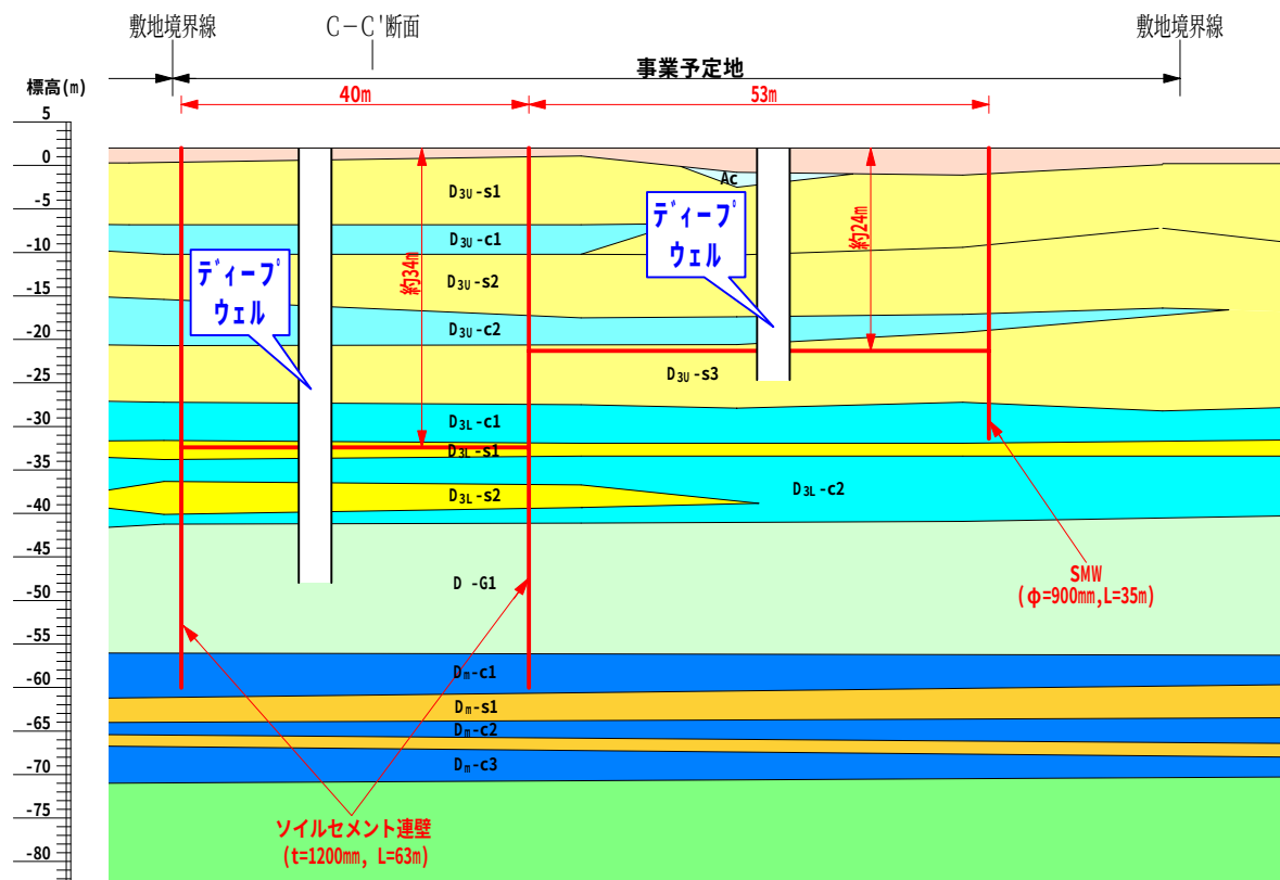
図 2-4-8 掘削時の山留壁及び排水計画
