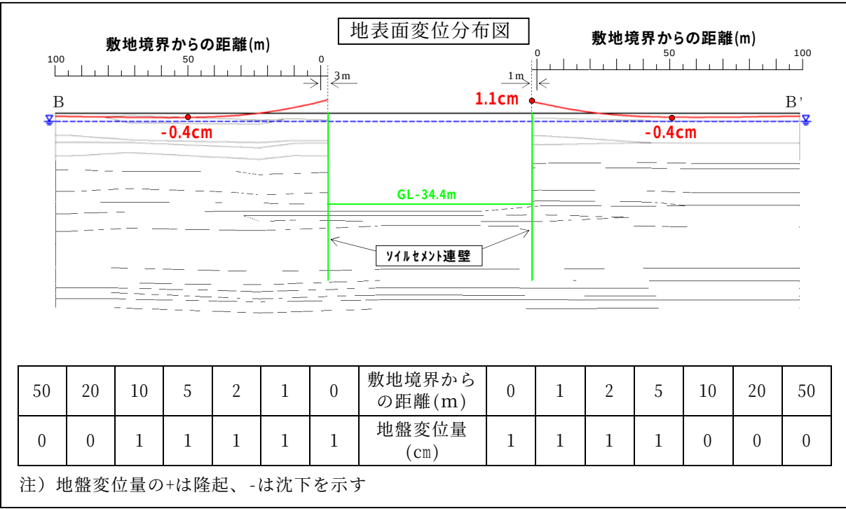
図 2-4-10(2) 掘削工事後の地盤変位 (B-B'断面)
