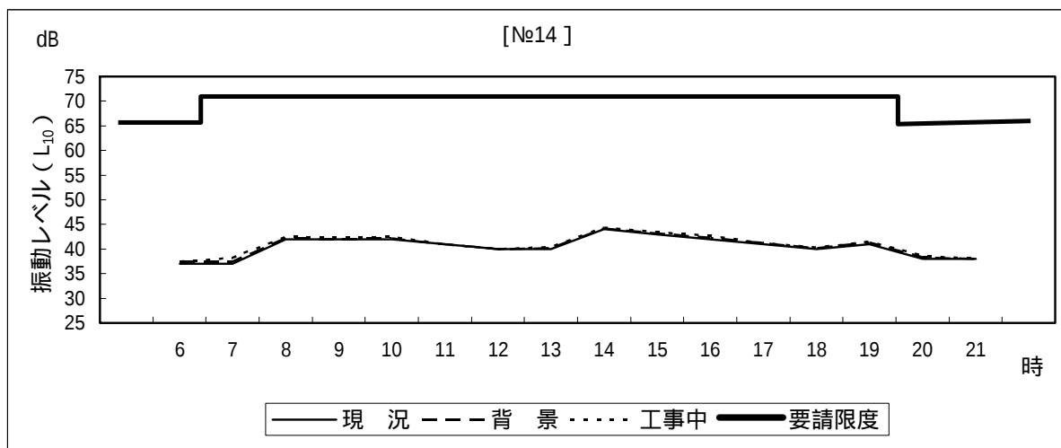
図2-3-6(4) 道路交通振動の振動レベル ( L_{10} ) 予測結果
