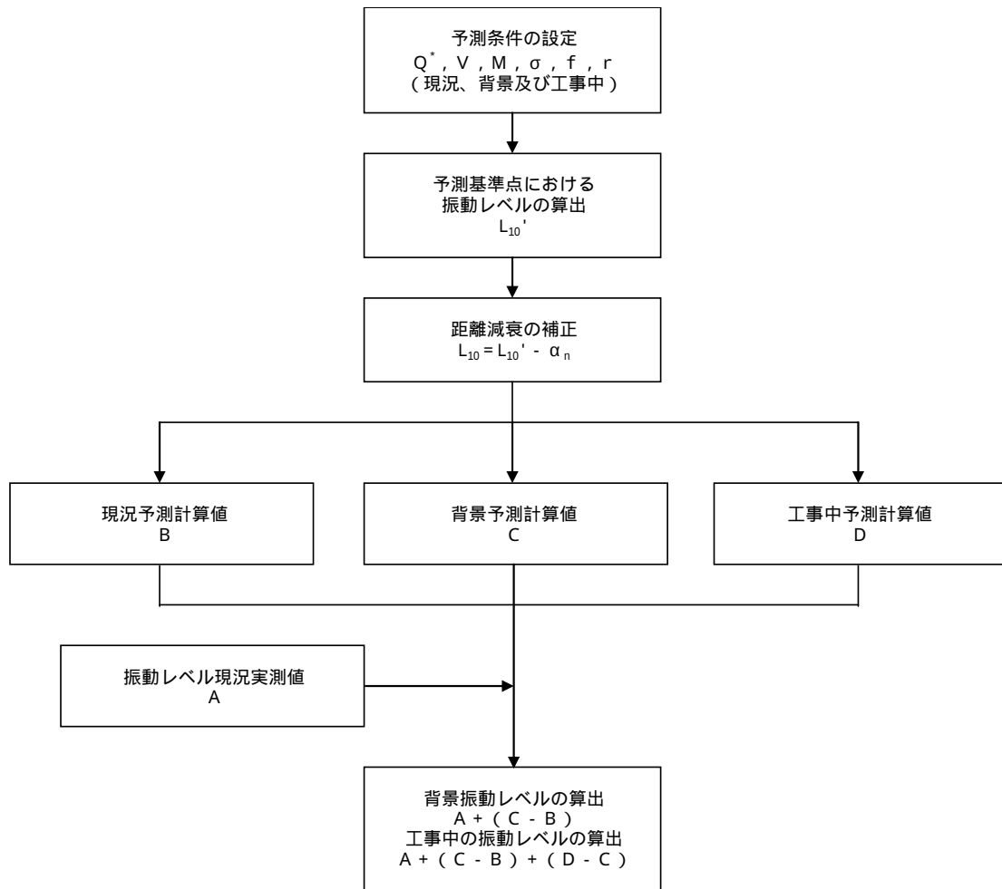
注) 図中の記号 ( Q^* 、 V 、 M 、 \sigma 、 f 、 r 、 L_{10} 、 L_{10}' 、 \alpha_n ) は、資料 5 - 7 (資料編 p.263) 参照 図 2-3-5 工事関係車両の走行による振動の予測手順 (旧建設省土木研究所の提案式)
