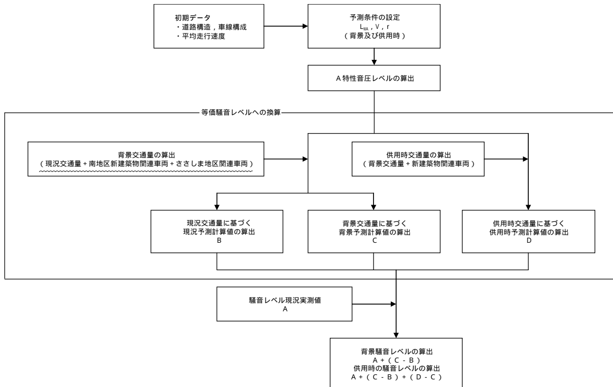
図 2-2-11 新建築物関連車両の走行による騒音の予測手順
