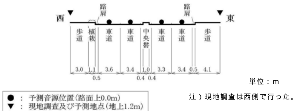
図 2-2-9(2) 音源配置図（道路断面方向の配置イメージ：No 4 の例）
