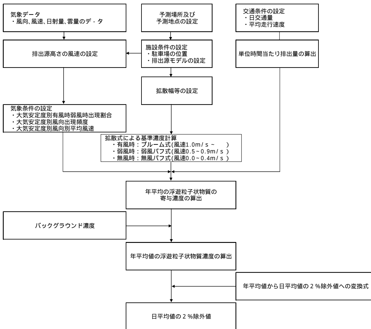
図 2-1-18 事業予定地内における駐車場の設置による浮遊粒子状物質の予測手順
