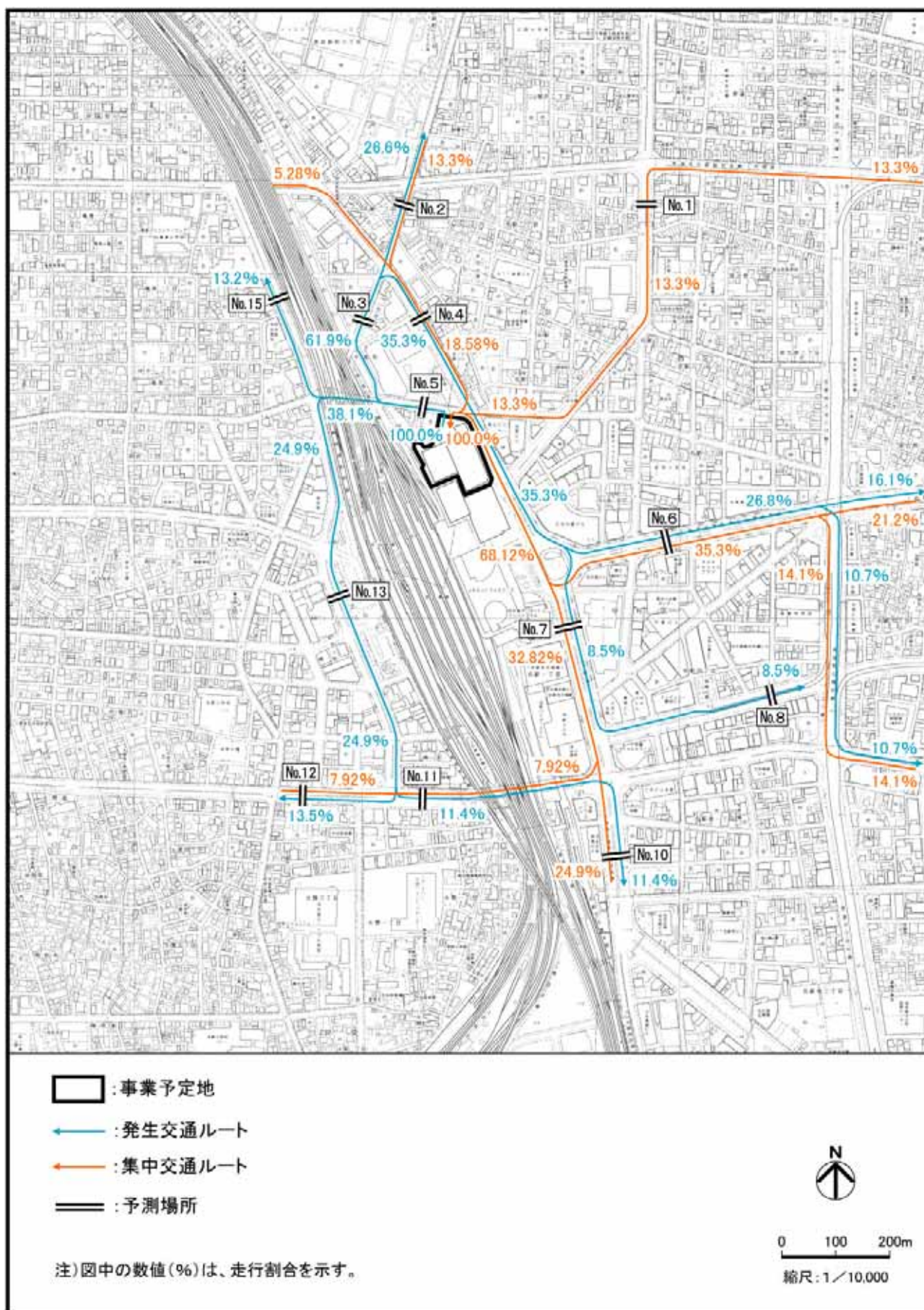
図 2-1-20 新建築物関連車両の走行ルート、走行割合及び予測場所
