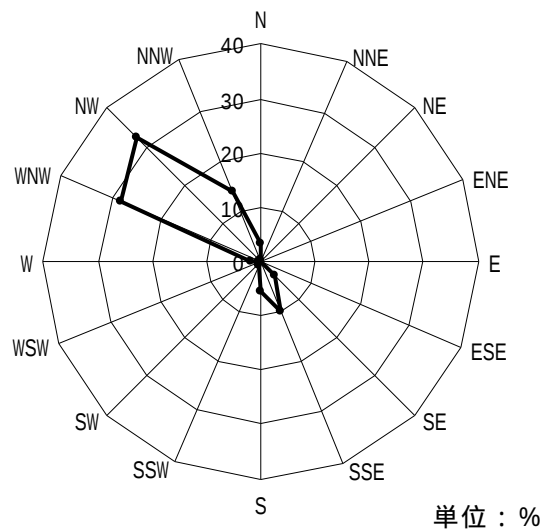
図 2-1-3 風力階級 4 以上による年間風配図 注) (地上 30m)
