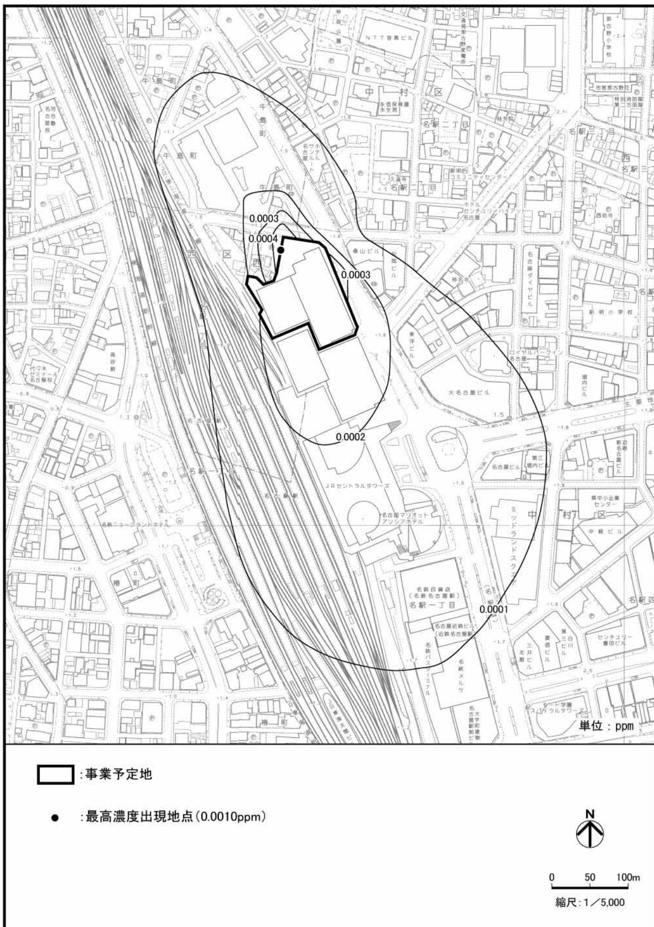
図 2-1-17 事業予定地内における駐車場の設置による二酸化窒素の予測結果
