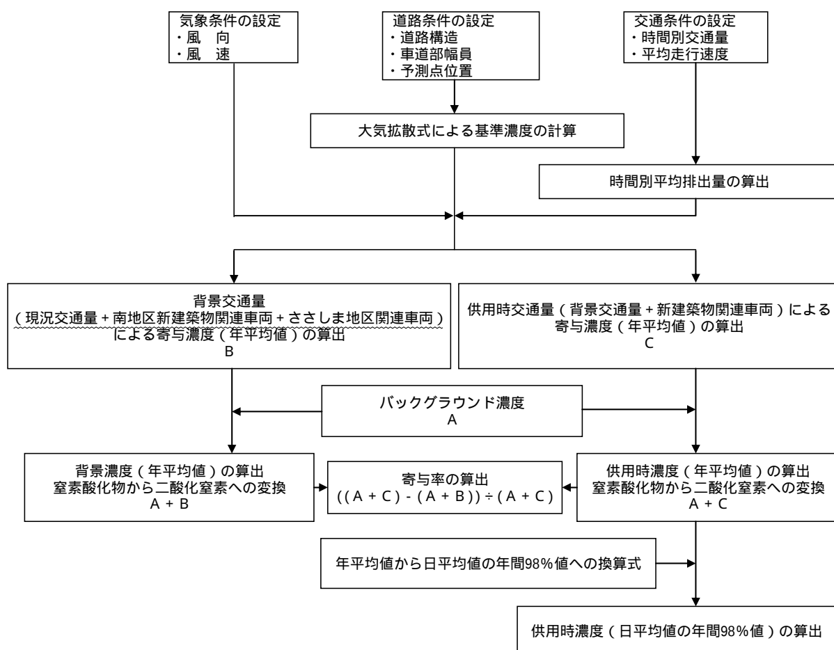
図 2-1-21 新建築物関連車両の走行による二酸化窒素の予測手順
