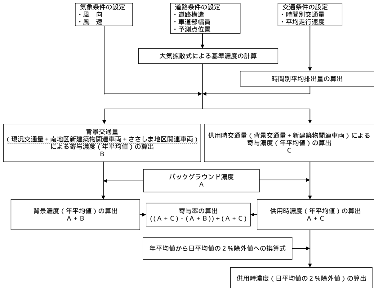
図 2-1-22 新建築物関連車両の走行による浮遊粒子状物質の予測手順
