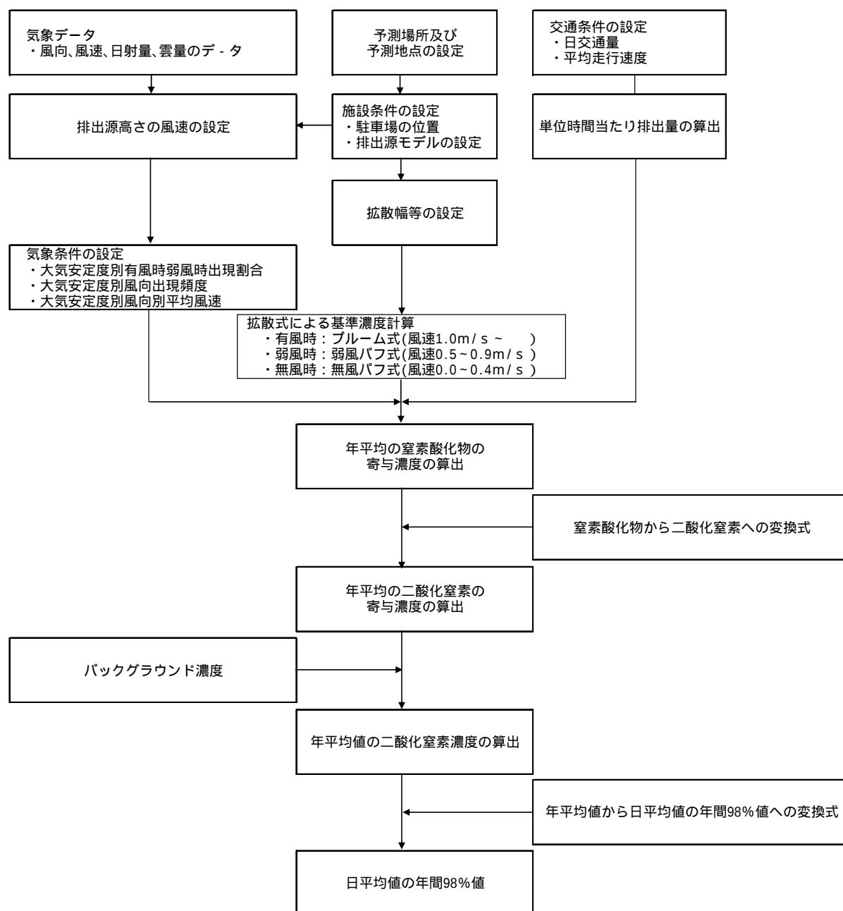
図 2-1-15 事業予定地内における駐車場の設置による二酸化窒素の予測手順
