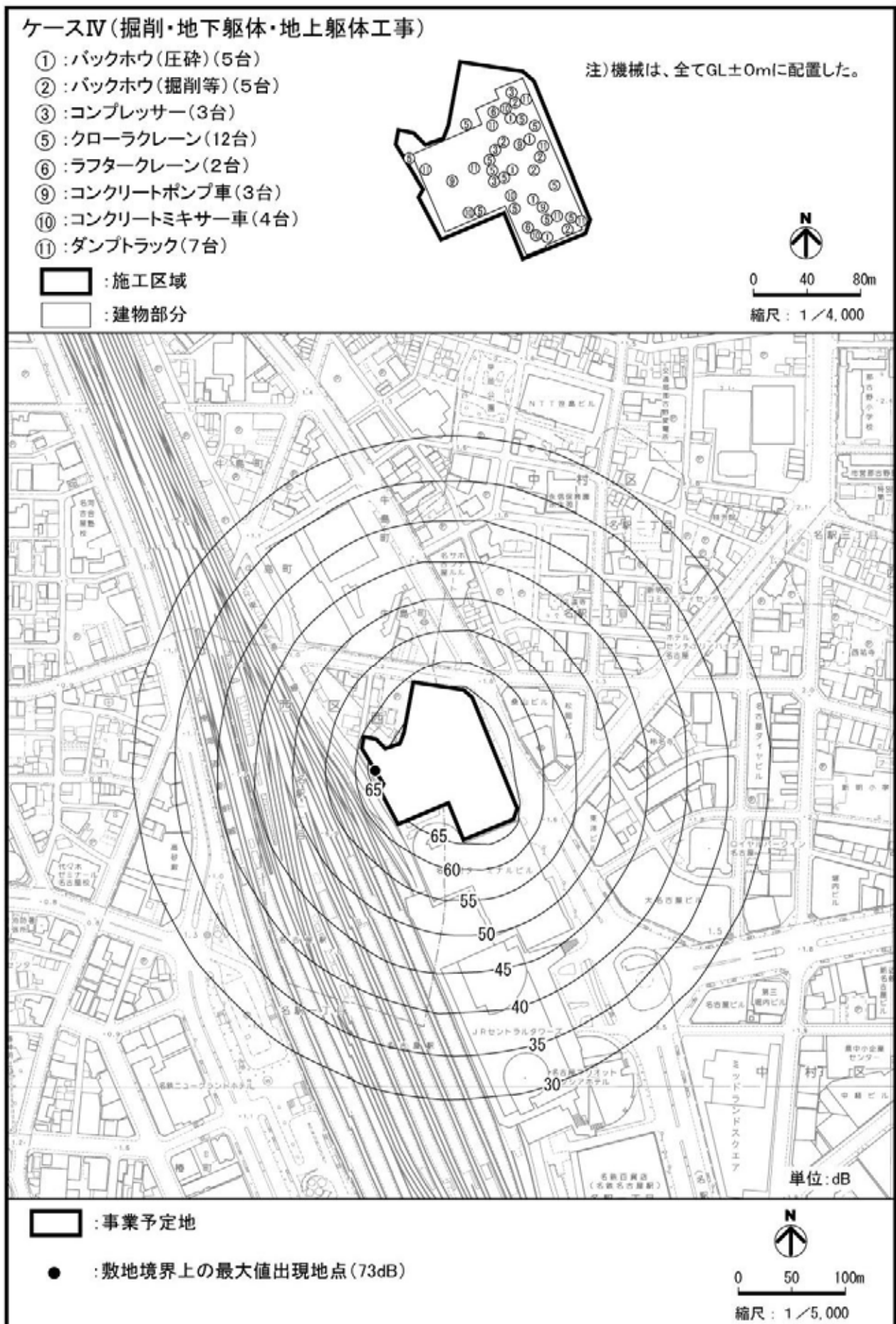
図 2-3-3(4) 建設機械の稼働による振動レベルの予測結果 (ケースⅣ)
