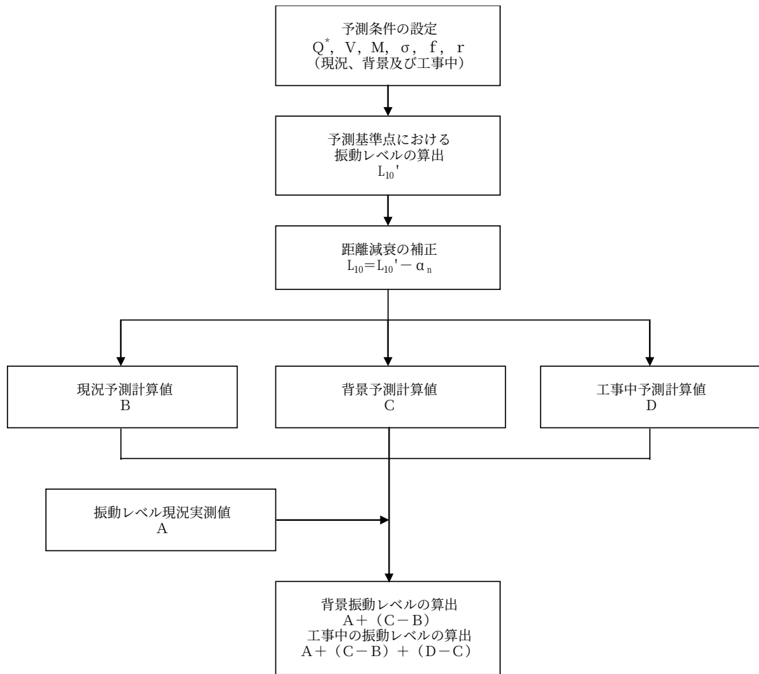
注) 図中の記号 ( Q^* 、 V 、 M 、 \sigma 、 f 、 r 、 L_{10} 、 L_{10}' 、 \alpha_n ) は、資料 5－6 (資料編 p.257) 参照 図 2-3-5 工事関係車両の走行による振動の予測手順 (旧建設省土木研究所の提案式)
