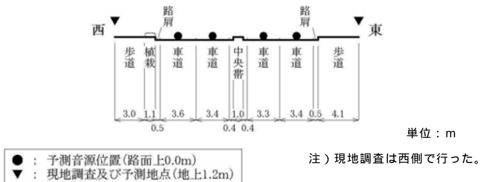
図 2-2-9(2) 音源配置図（道路断面方向の配置イメージ：№ 4 の例）
