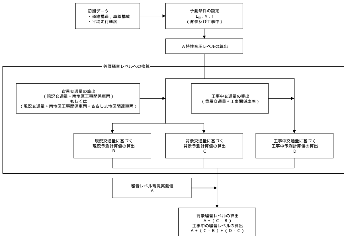
図 2-2-8 工事関係車両の走行による騒音の予測手順
