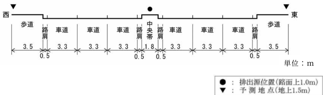
図 2-1-15(2) 点煙源の位置 (No.3 断面の例)
