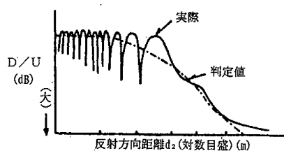
反射方向中心線のDU比
