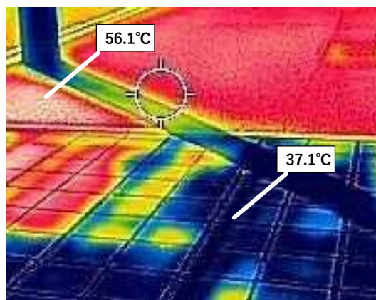
保水性ブロック舗装 (B) の写真 (左) とサーモカメラ画像 (右) 撮影日：8月29日 (送水時間：6min/h)
