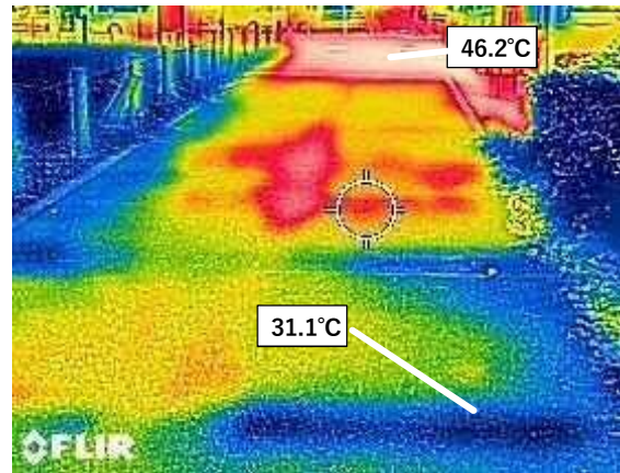
保水性アスファルト舗装 (A) の写真 (左) とサーモカメラ画像 (右) 撮影日：7月11日 (送水時間：40min/h)
