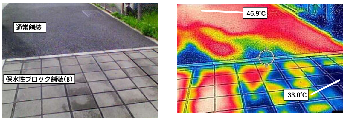
保水性ブロック舗装 (B) の写真 (左) とサーモカメラ画像 (右) 撮影日：8月10日 (送水時間：6min/h)
