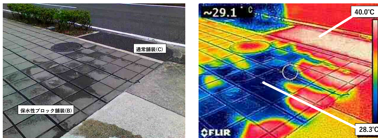
保水性ブロック舗装 (B) の写真(左)とサーモカメラ画像(右) 撮影日：7月2日 (送水時間：4min/h)
