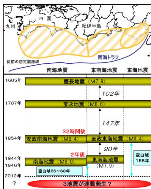
図1.1.1 南海トラフ沿い地震の発生時期と領域
