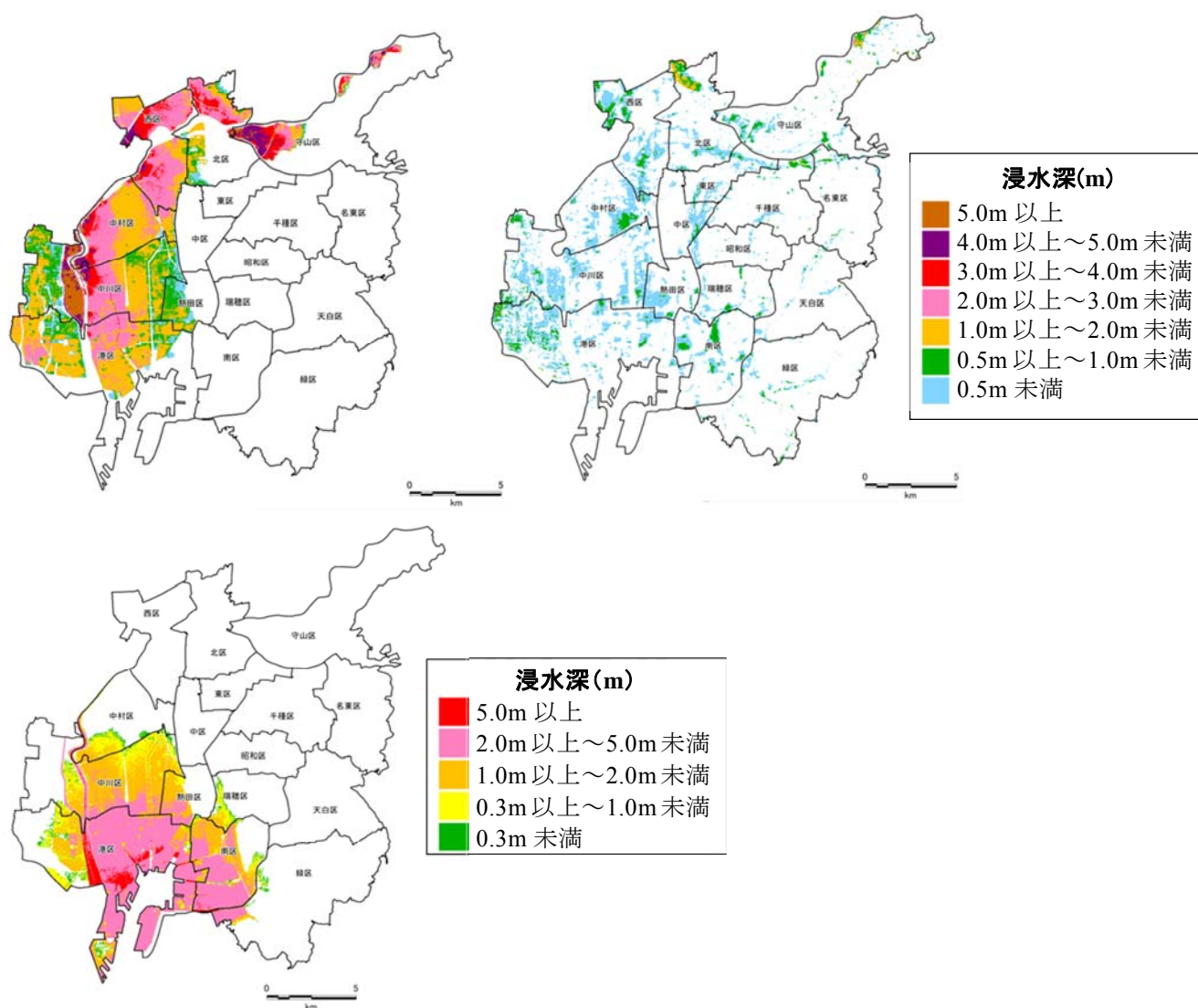
図 1.1.4 浸水範囲・浸水深（上段左：洪水、上段右：内水氾濫、下段：高潮）
