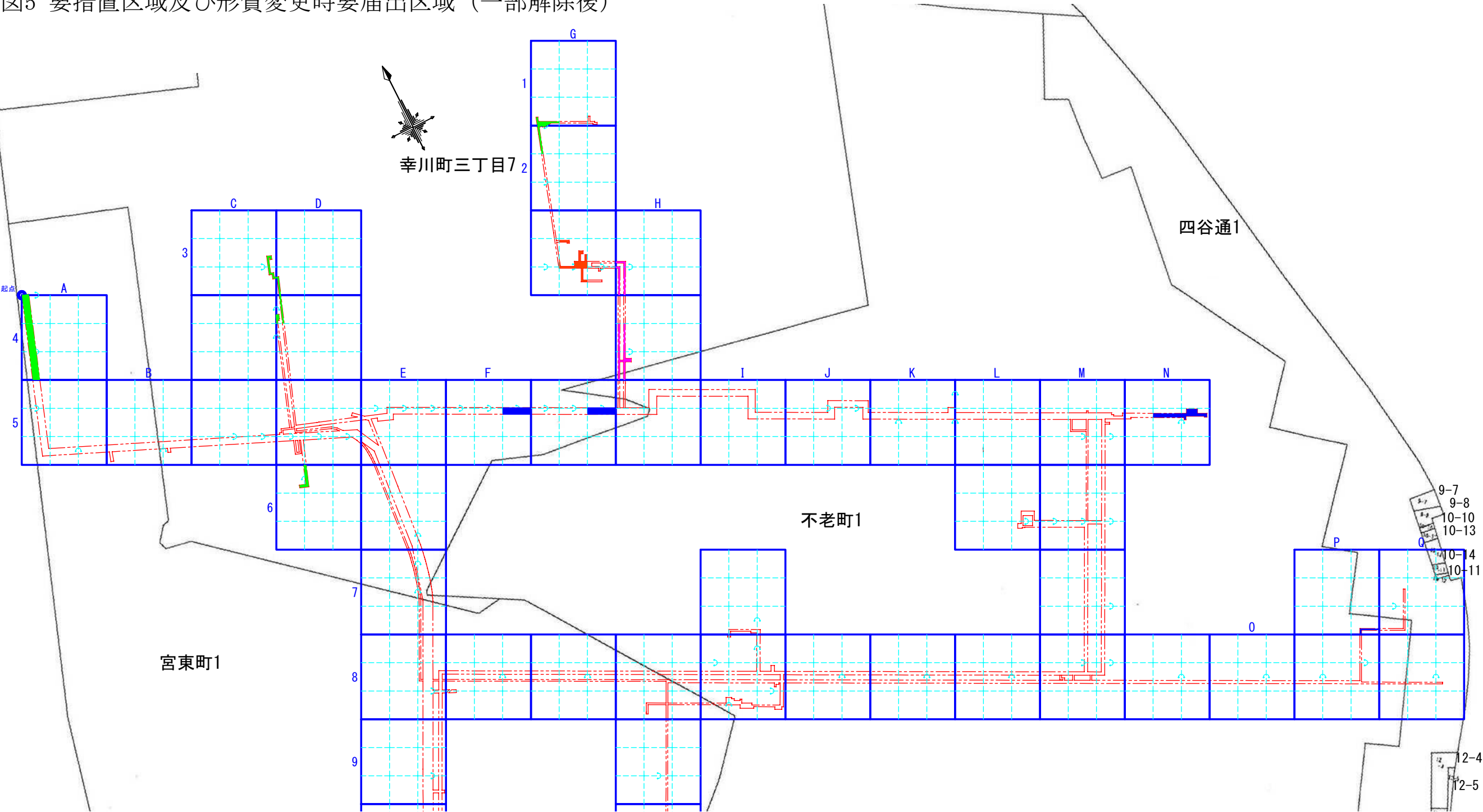
図5 要措置区域及び形質変更時要届出区域（一部解除後）
