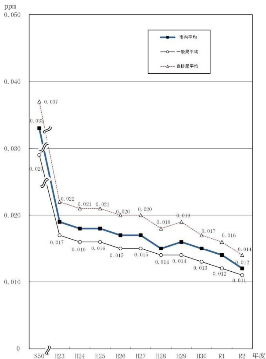
図 3-2-1 二酸化窒素年平均値の推移
