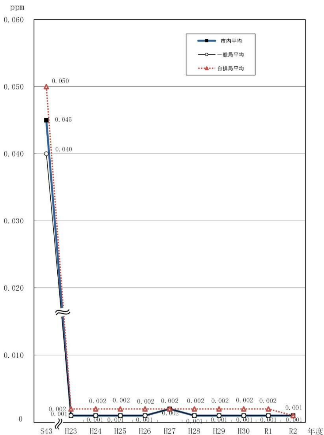
図 3-1-1 二酸化硫黄年平均値の推移
