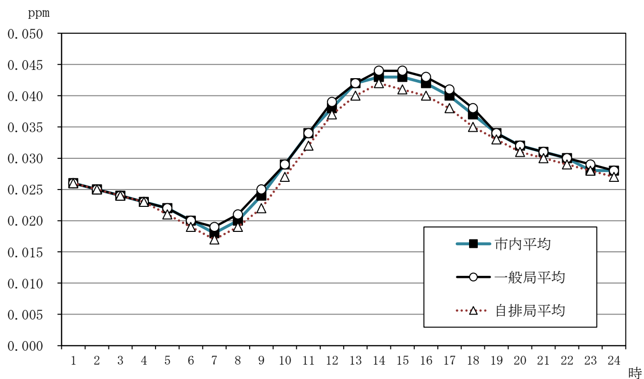
図 3-5-3 光化学オキシダント時刻別平均濃度の市内平均(令和2年度)
