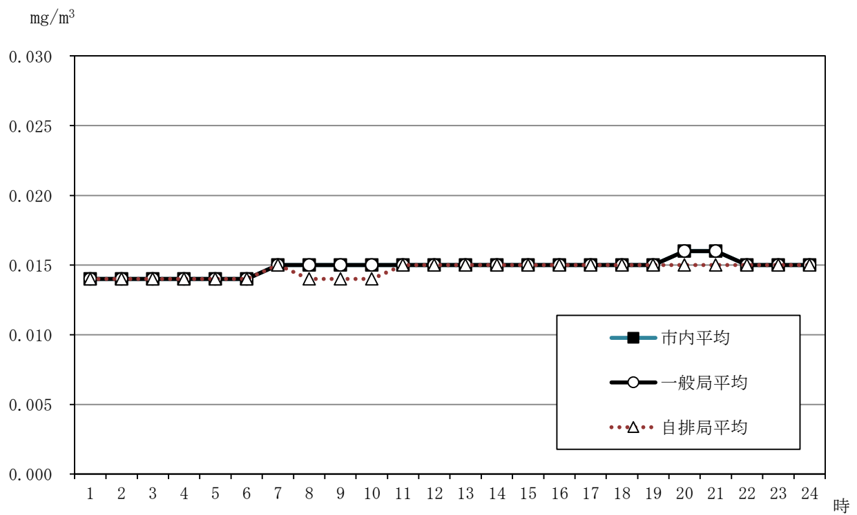
図 3-4-3 浮遊粒子状物質時刻別平均濃度の市内平均（令和 2 年度）
