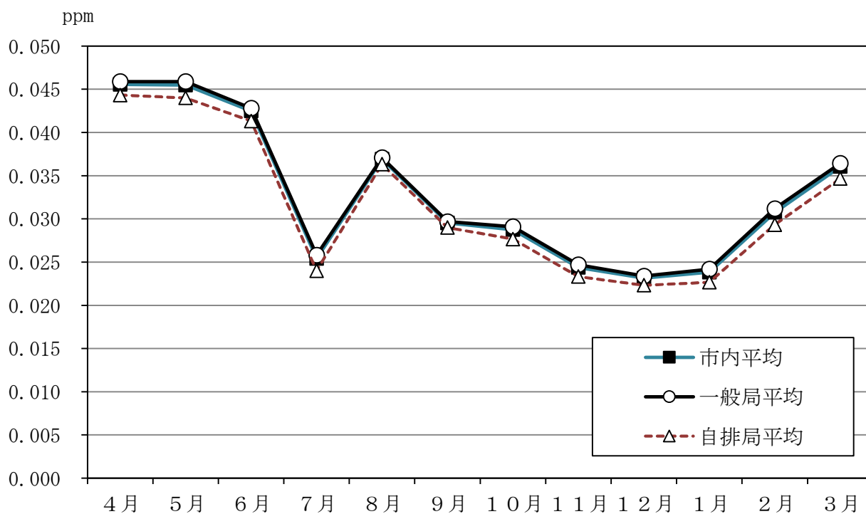
図 3-5-2 光化学オキシダント昼間(5時～20時)月平均値の市内平均経月変化(令和2年度)
