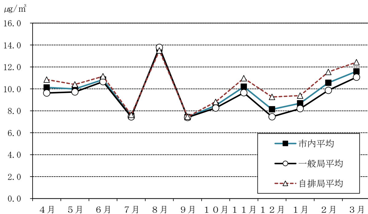
図 3-7-2 微小粒子状物質月平均値の市内平均経月変化（令和 2 年度）
