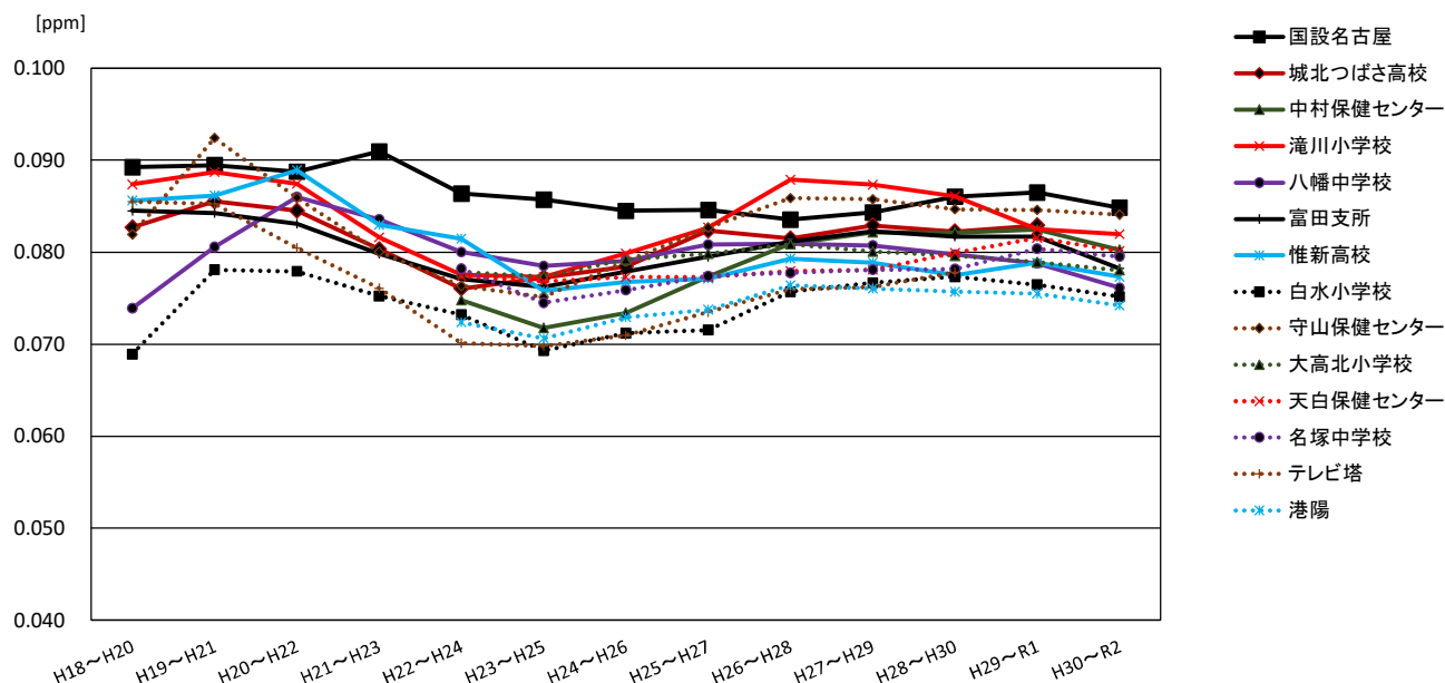
図 3-5-4 日最高 8 時間値の年間 99 パーセンタイル値の 3 年移動平均値の経年変化
