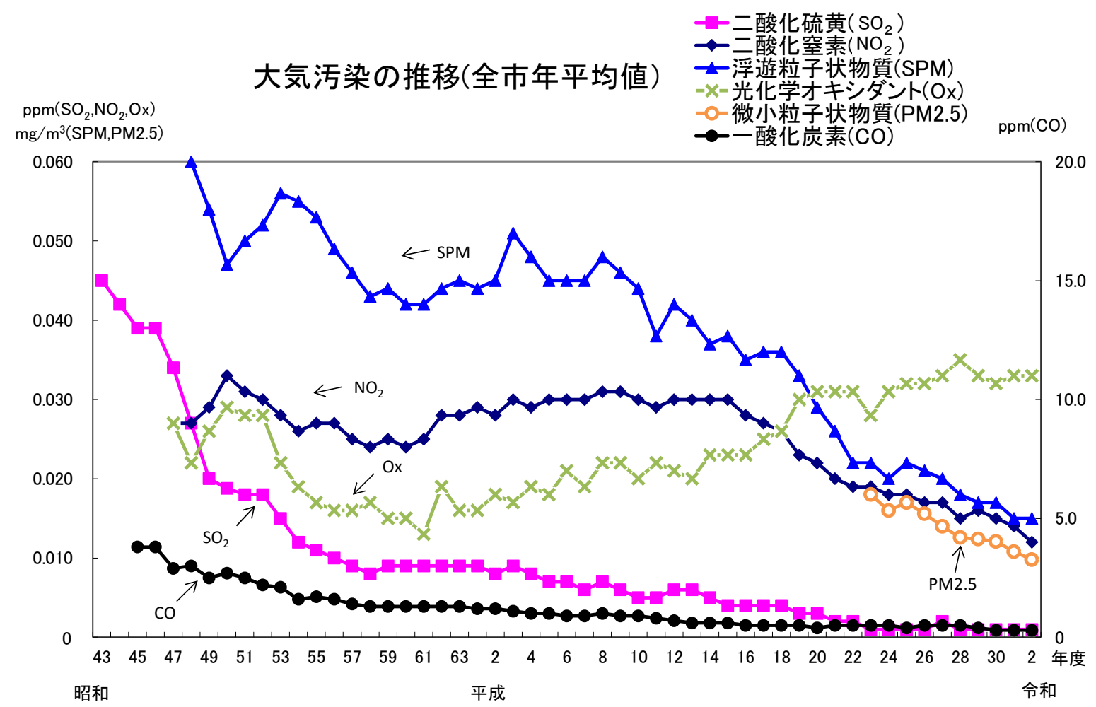
図 1 大気汚染の推移 (年平均値の市内平均)
