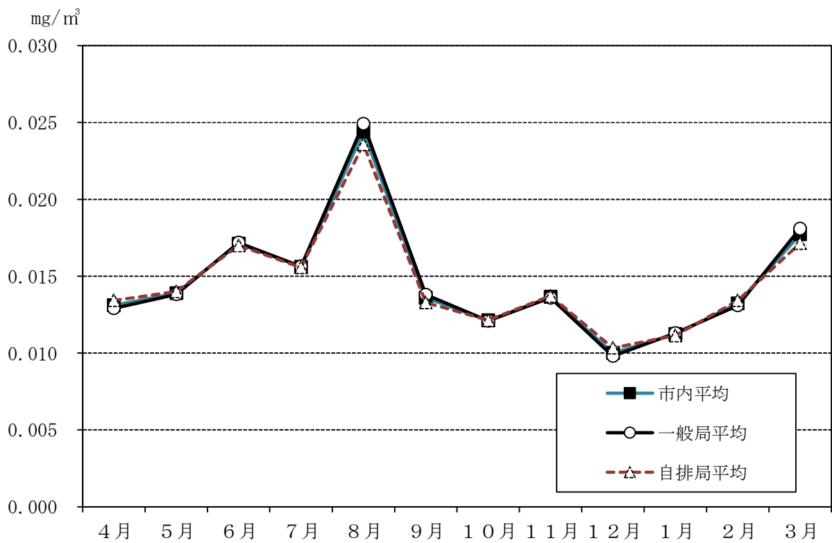
図 3-4-2 浮遊粒子状物質月平均値の市内平均経月変化（令和 2 年度）
