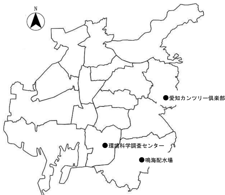
図 4-1 酸性降下物測定地点
