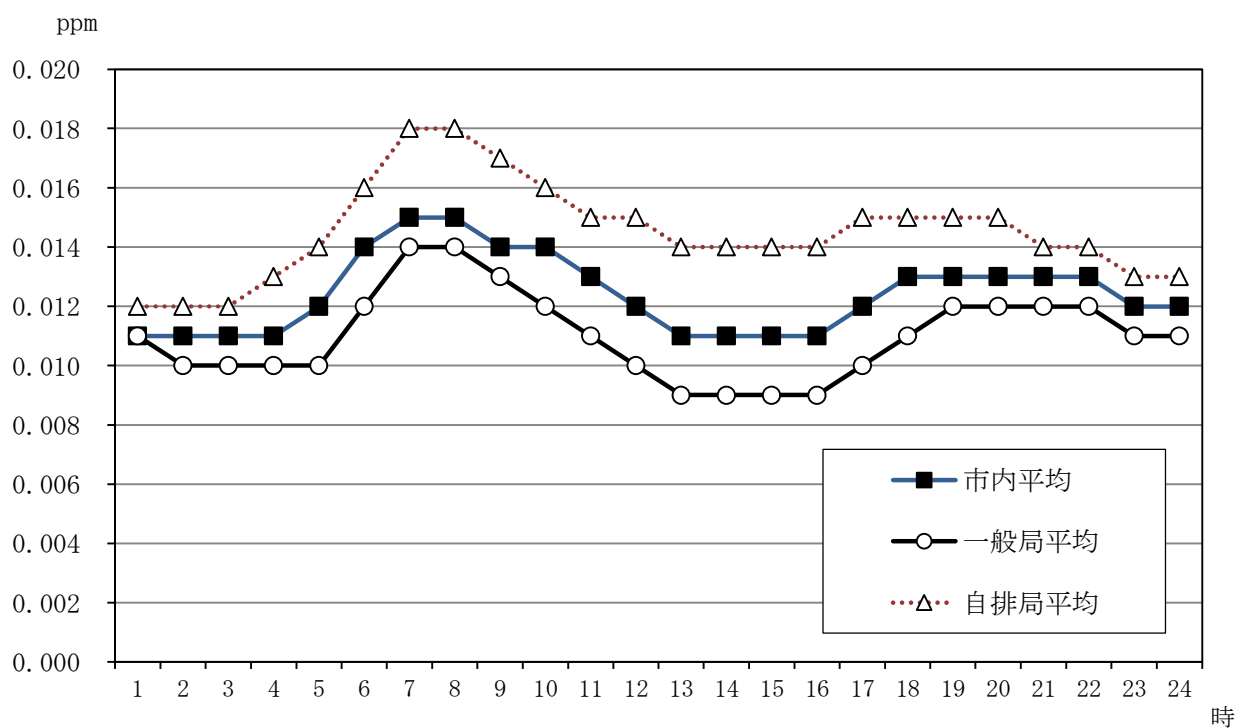
図 3-2-3 二酸化窒素時刻別平均濃度の市内平均（令和2年度）
