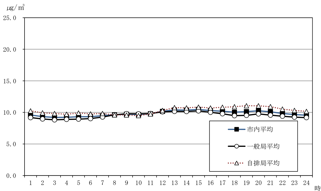
図 3-7-3 微小粒子状物質時刻別平均濃度の市内平均（令和 2 年度）
