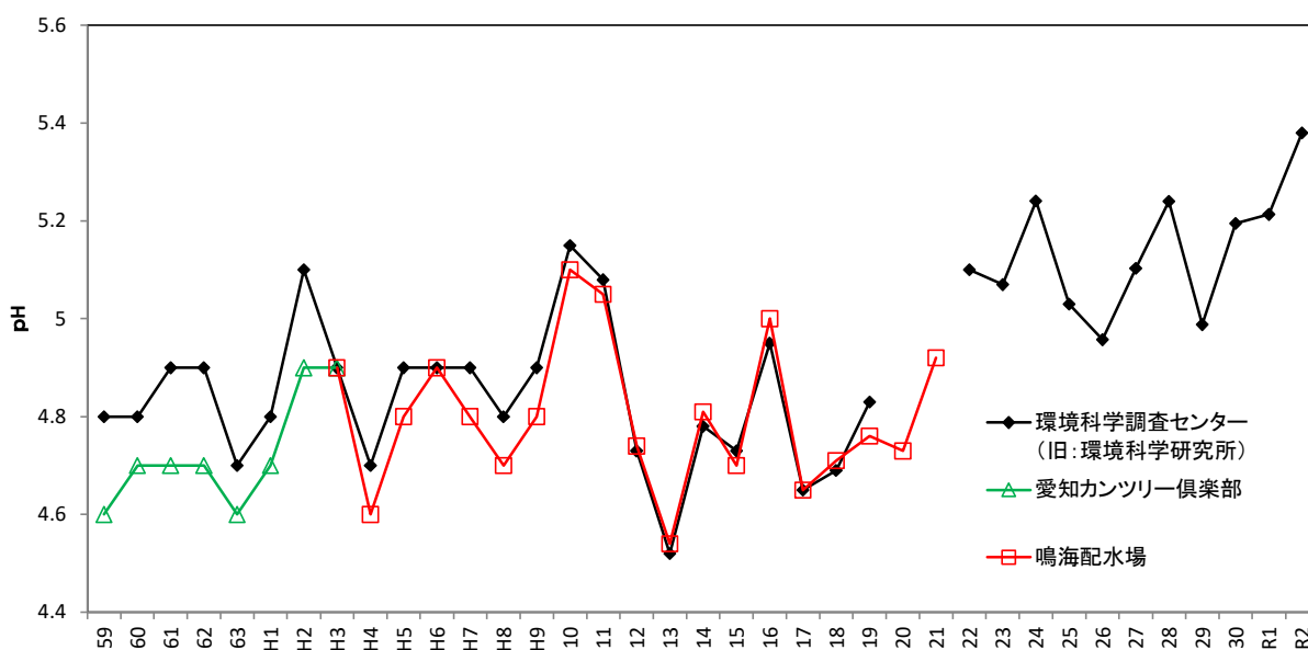
図 4-2 湿性降下物の pH 年平均値の推移
