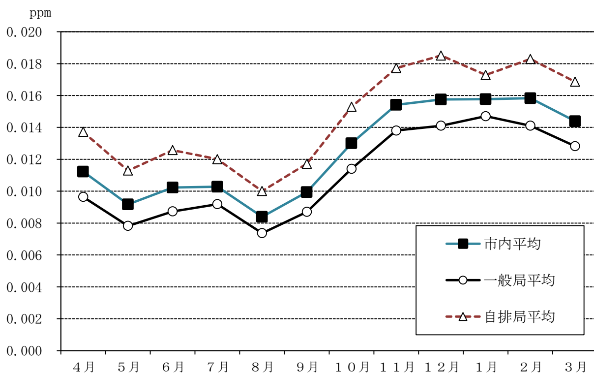
図 3-2-2 二酸化窒素月平均値の市内平均経月変化（令和2年度）
