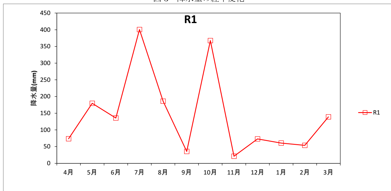
図4 月別降水量
