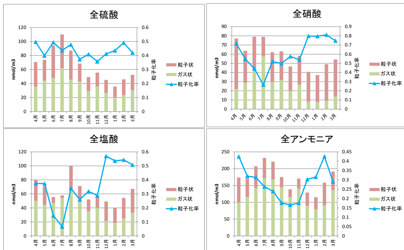
図 14 全硫酸、全硝酸、全塩化物、全アンモニア濃度の経月変化 (令和元年度)
