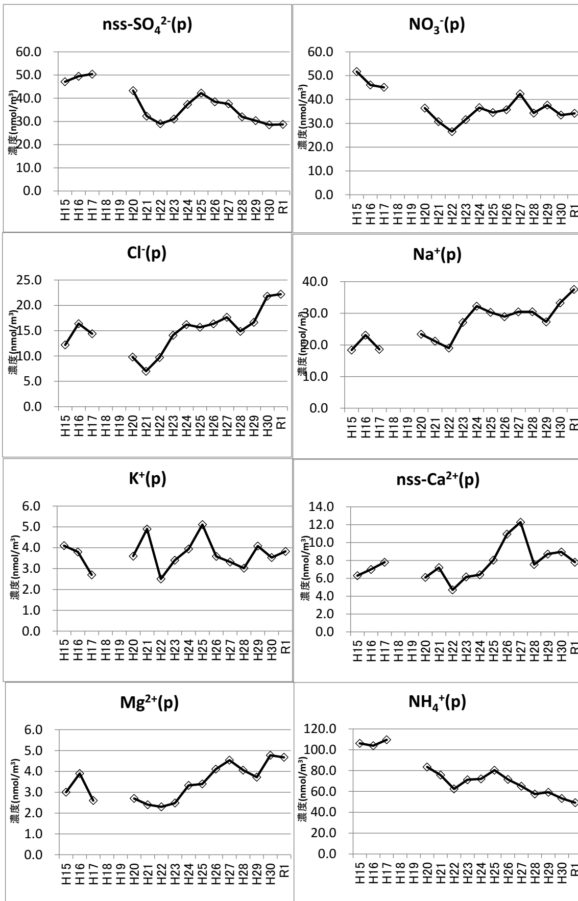
図 12 粒子状成分の経年変化
