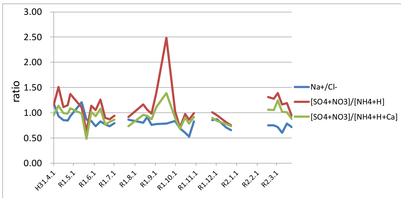
図8 イオン成分のバランスについて
