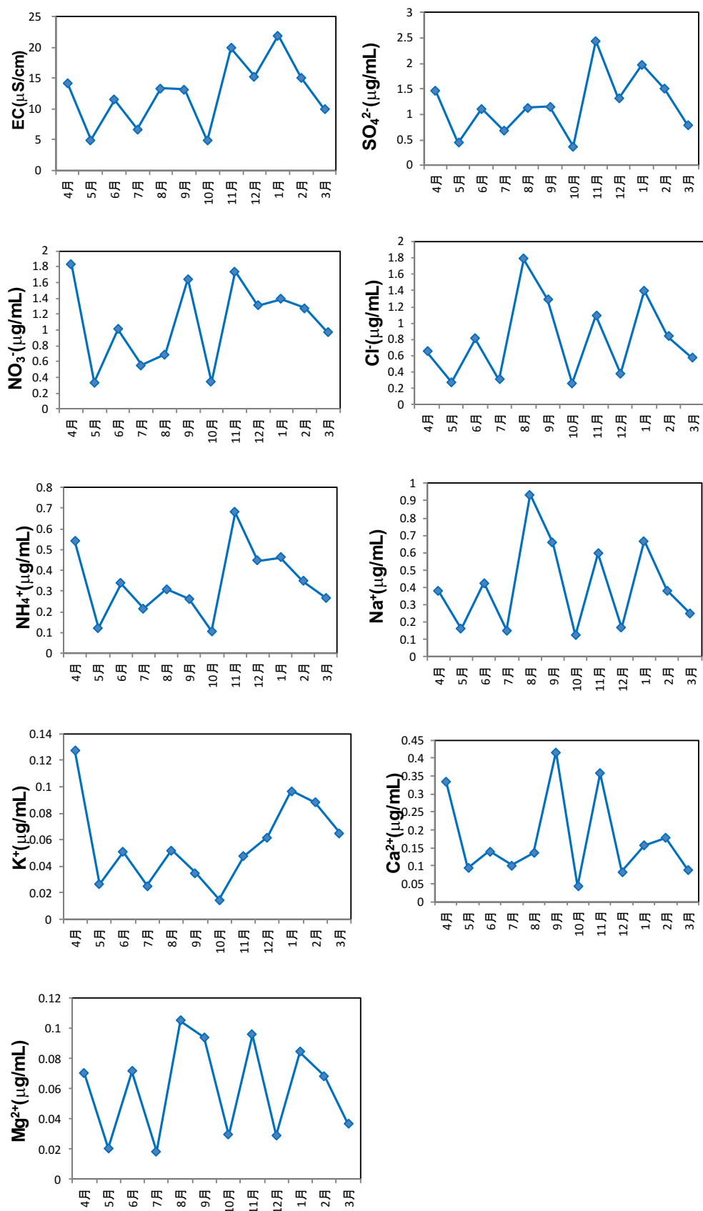
図7 加重月平均値の経月変化
