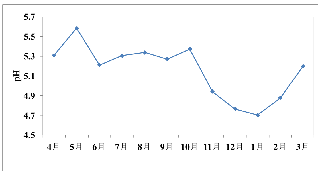
図 6 加重平均 pH 値の経月変化
