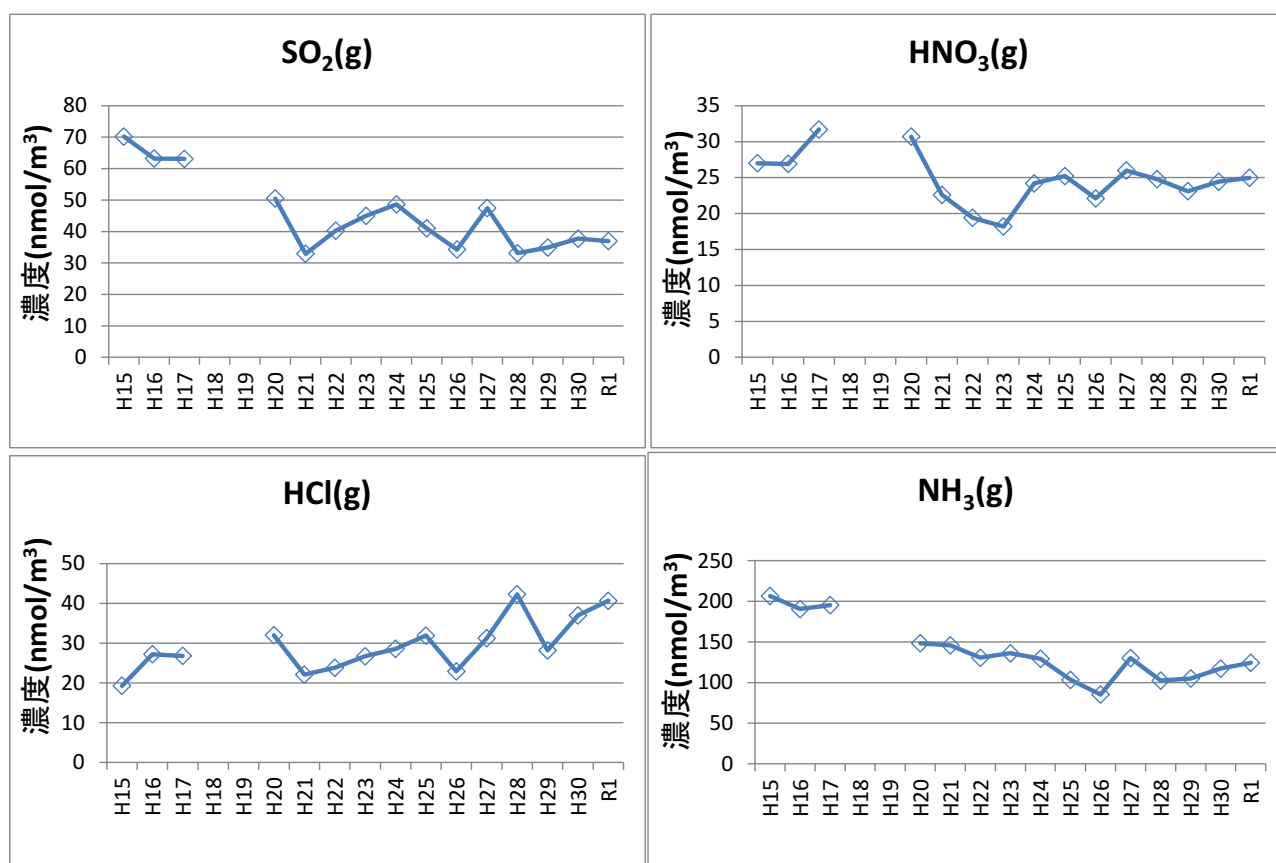
図 10 ガス状成分の経年変化
