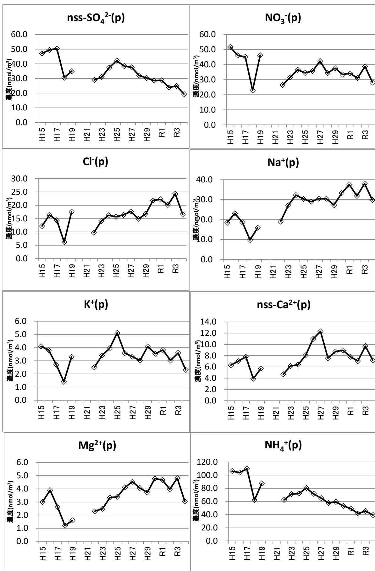
図 12 粒子状成分の経年変化
