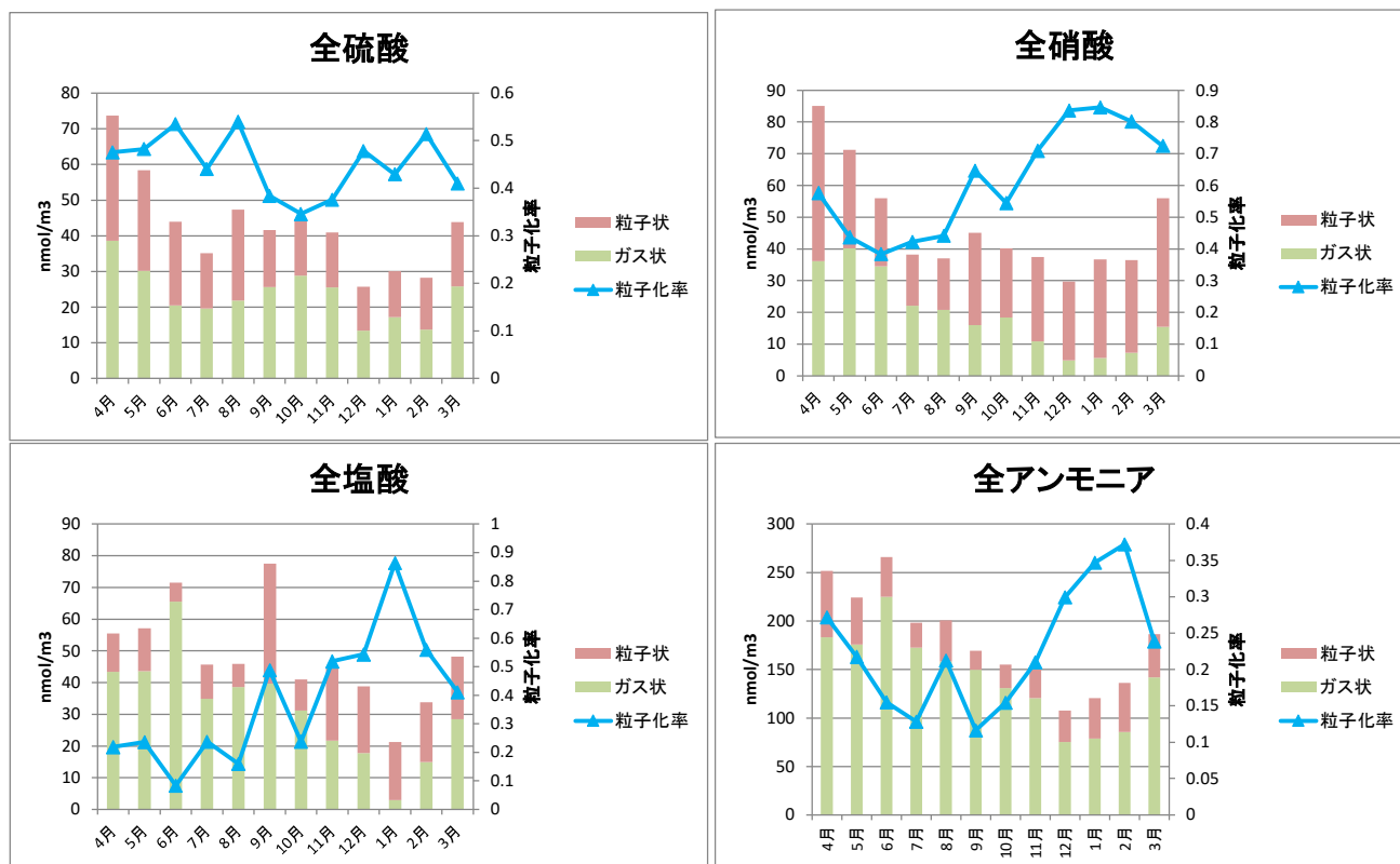
図 14 全硫酸、全硝酸、全塩化物、全アンモニア濃度の経月変化 (令和 4 年度)
