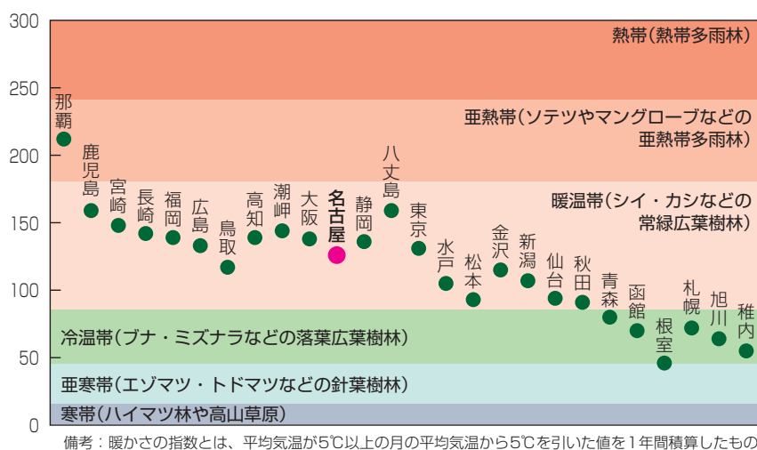
暖かさの指数と気候帯
