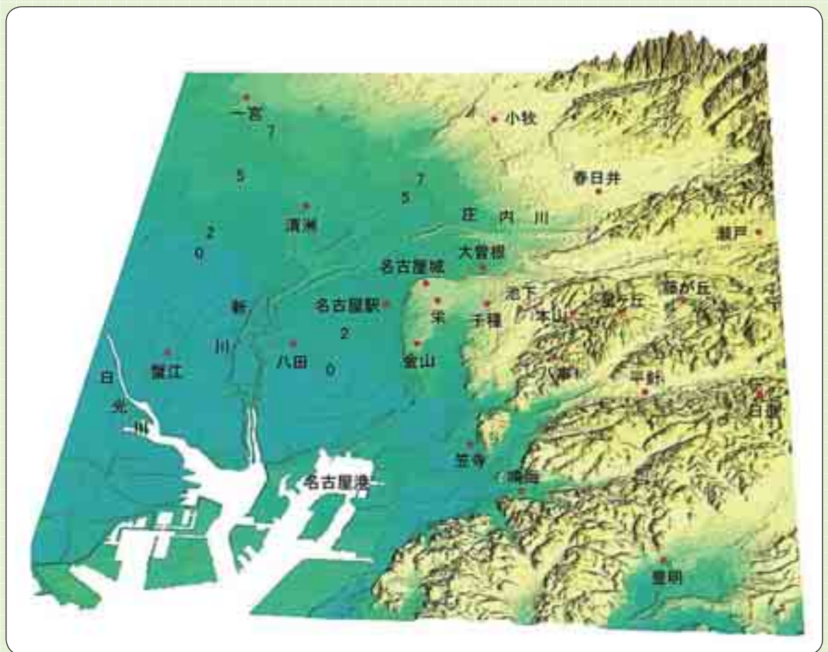
出典：新修名古屋市史 資料編 自然(名古屋市 平成20年) 備考：数字は標高値m
