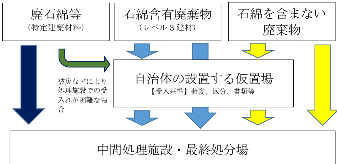
図8. 1 石綿に係る廃棄物の区分ごとの取り扱いフロー
