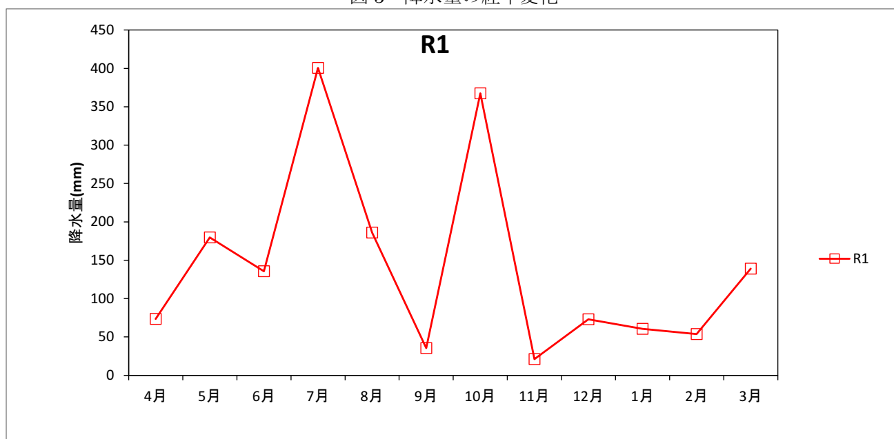
図4 月別降水量
