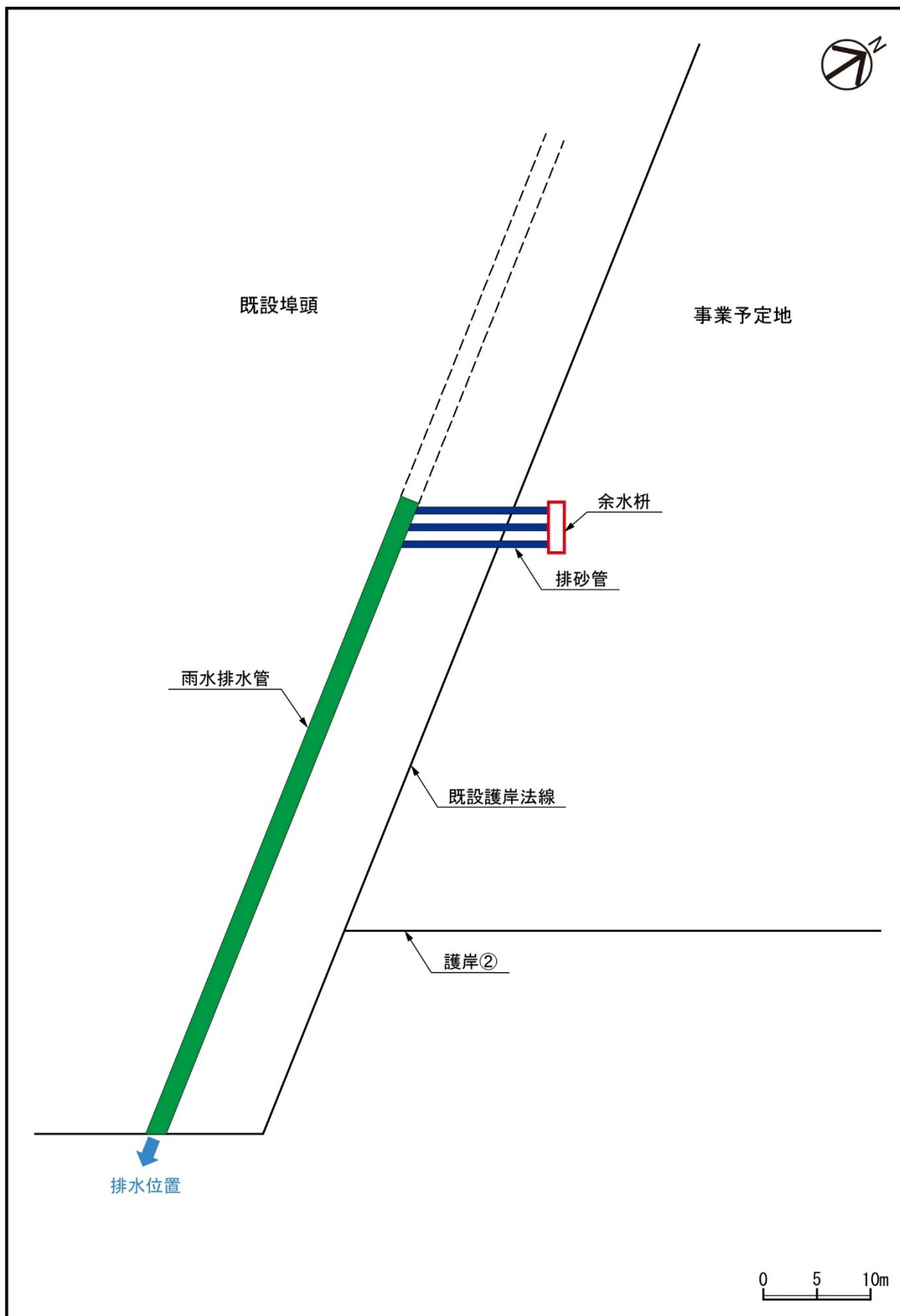
図 1-3-8 余水吐の構造図（平面図）
