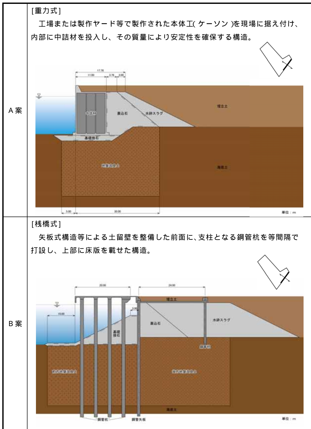
図 2-4-2 標準断面図
