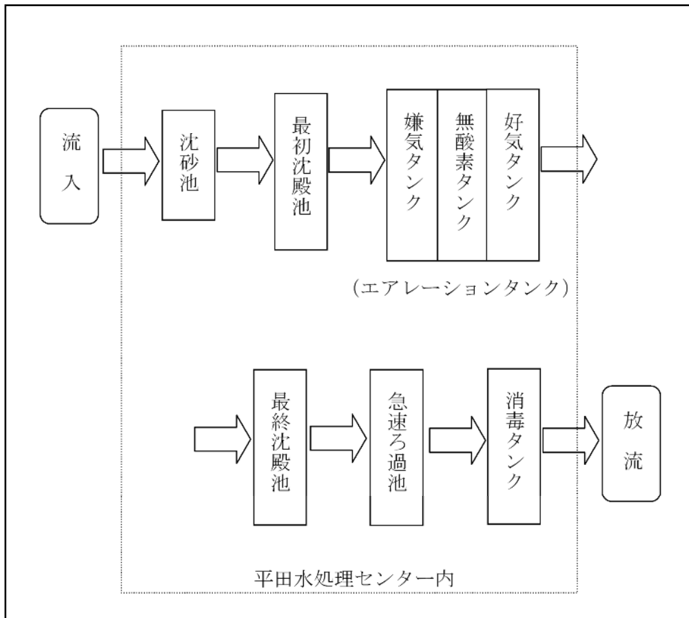
図 3-2 処理フロー
