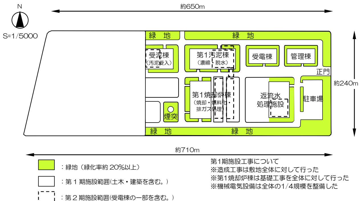
図 3-2 第 1 期及び第 2 期施設配置
