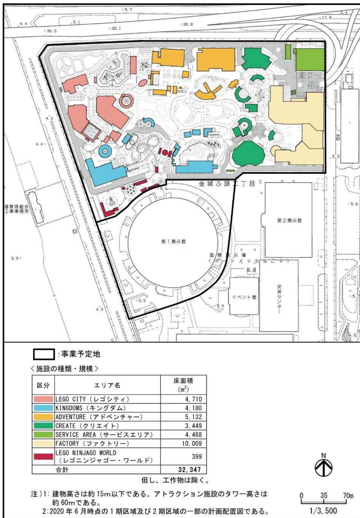
図 1-3-3(2) 計画配置図 (1期区域及び2期区域の一部)
