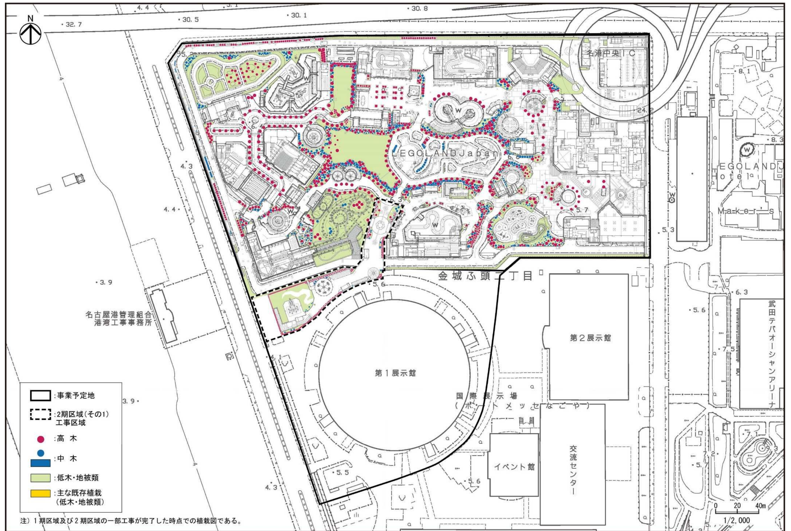
図 1-3-4(2) 緑化計画図 (1期区域及び2期区域の一部)
