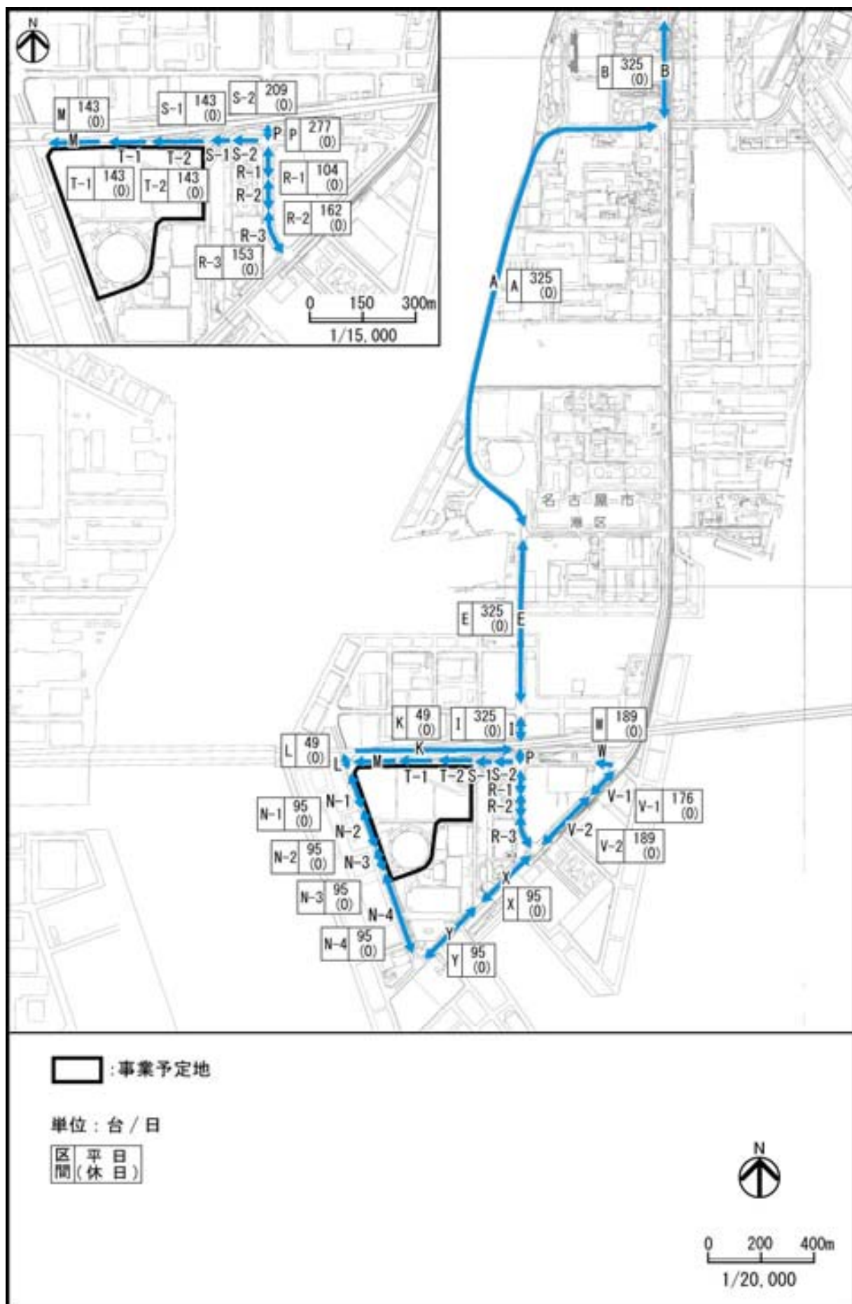
図－3(1) 商業施設等工事関係車両の区間断面交通量（1期区域工事着工後12ヶ月目）
