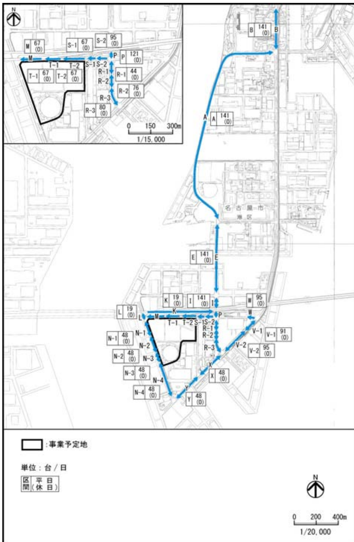
図－3(2) 商業施設等工事関係車両の区間断面交通量（1期区域工事着工後14ヶ月目）
