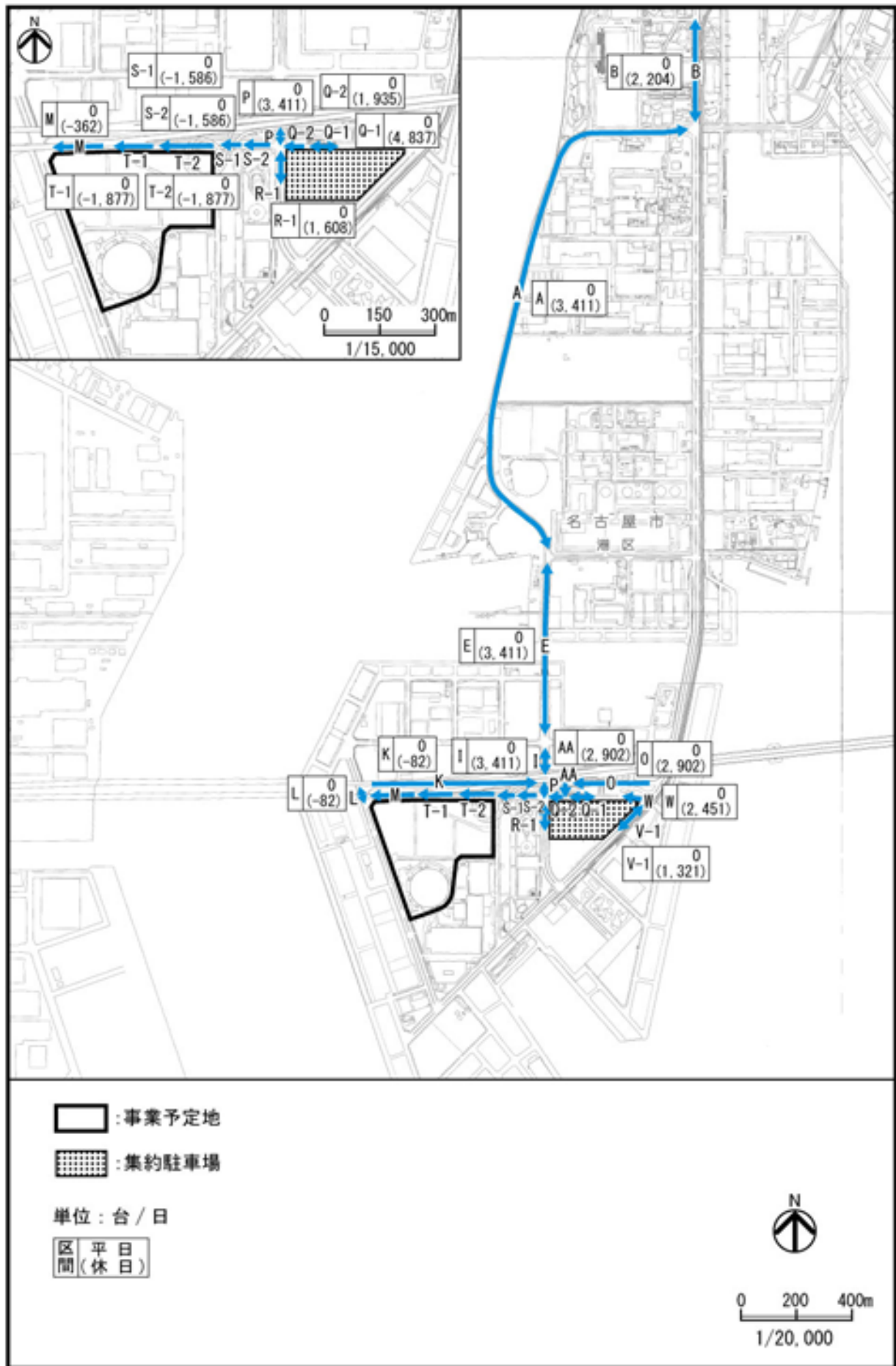
図－５（２） 集約駐車場への移行による国際展示場利用車両の区間断面交通量の増減
