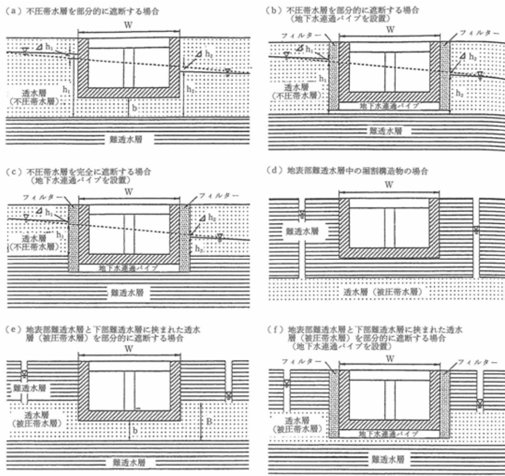
図 10-3 掘削構造物における地下水保全対策工
