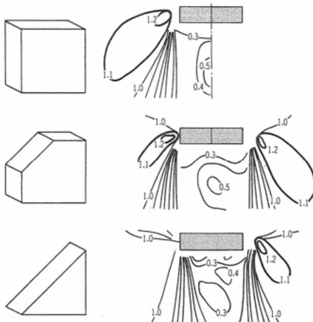
図 3-5 セットバックによる風速増加領域の変化
