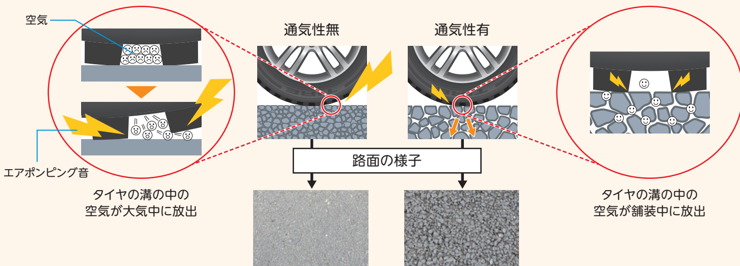
図3 通気性を持たない舗装(左図)と持つ舗装(右図) 通気性を持つ舗装が低騒音舗装
