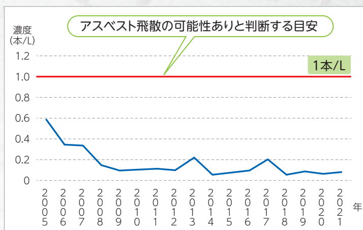
図4 アスベスト環境濃度(年平均値)の推移
