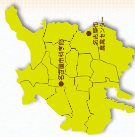
図7 CO2観測地点
