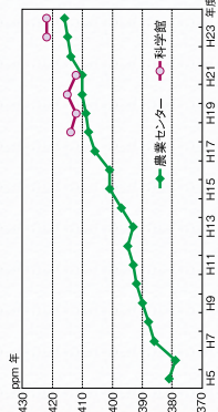
図6 CO2濃度年平均値の推移
