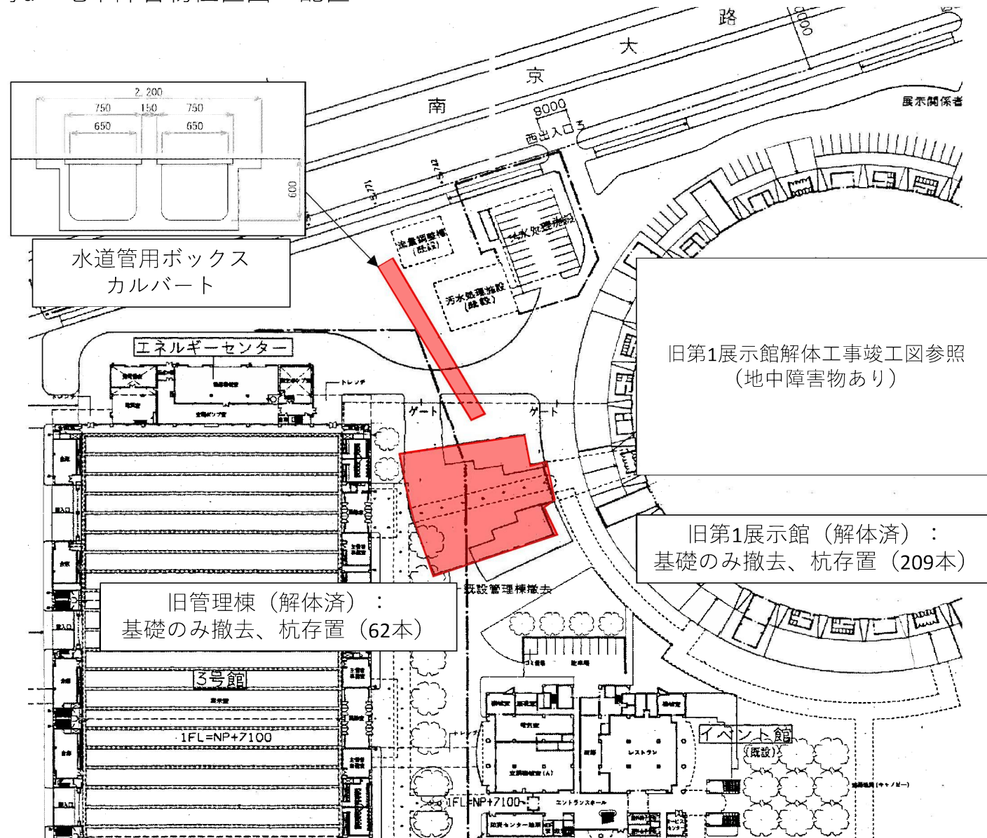
参考d 地中障害物位置図<配置>
