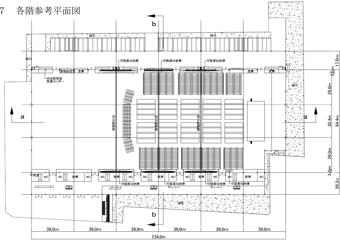
1階平面図 S=1/2000
