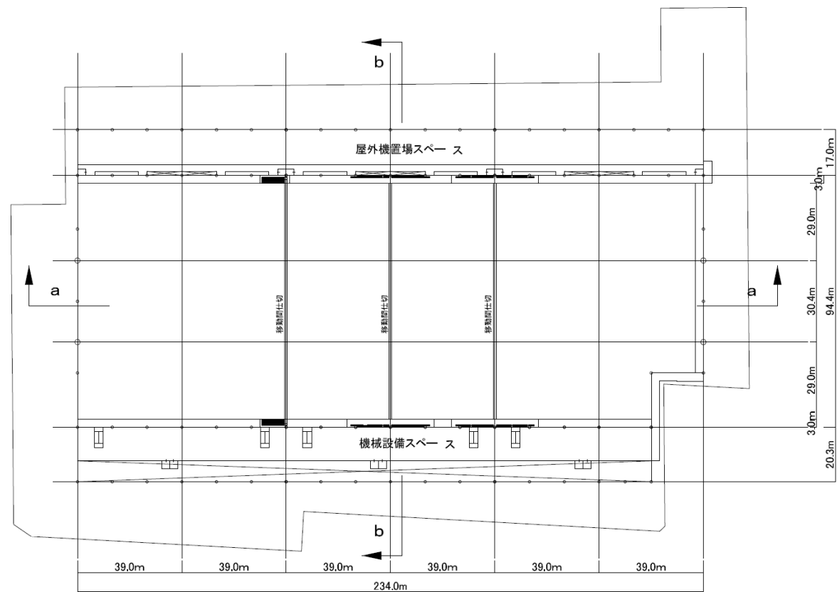
3階平面図 S=1/2000
