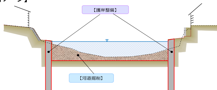
河道掘削状況 (尾頭橋上流)
