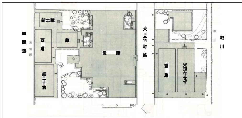
図 2-27 伊藤家住宅平面図
