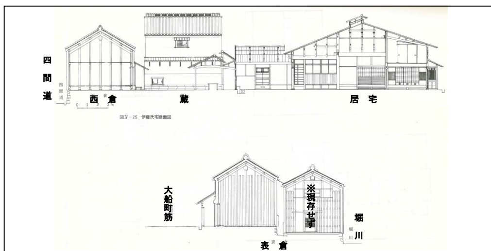
図 2-28 伊藤家住宅断面図
