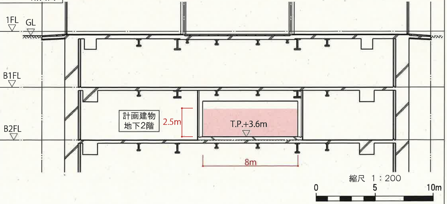
B-B' 断面図
