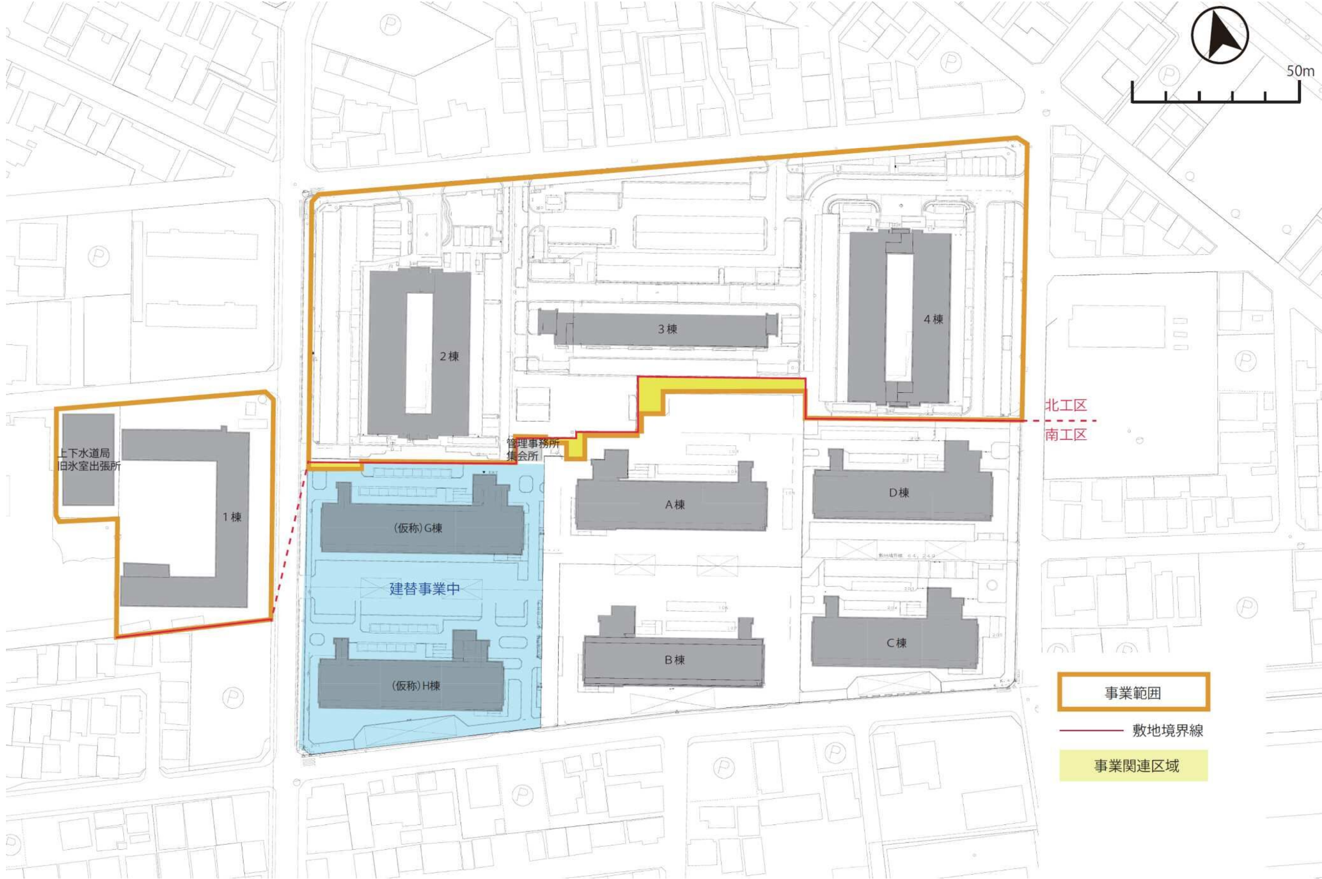
添付資料2 事業用地現況図 scale:1/1000
