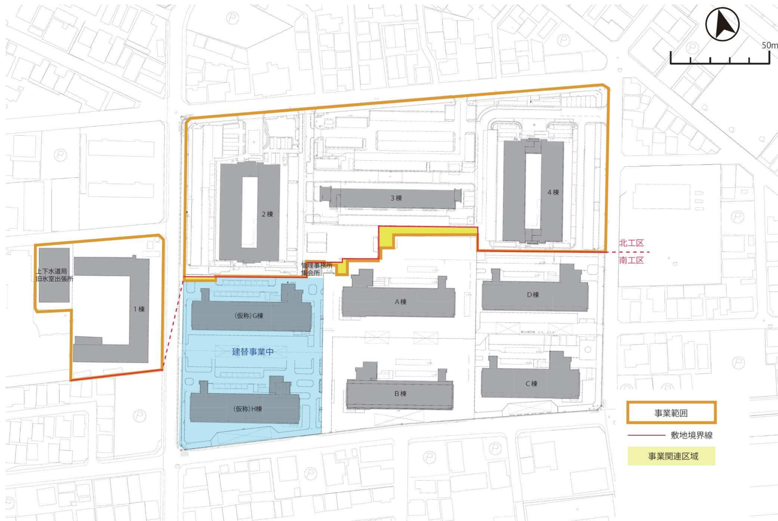
(別紙-3) 事業用地現況図 scale:1/1000
