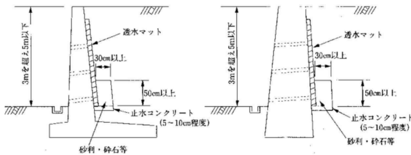
(b) 擁壁の見かけ高さが 3m を超える場合
