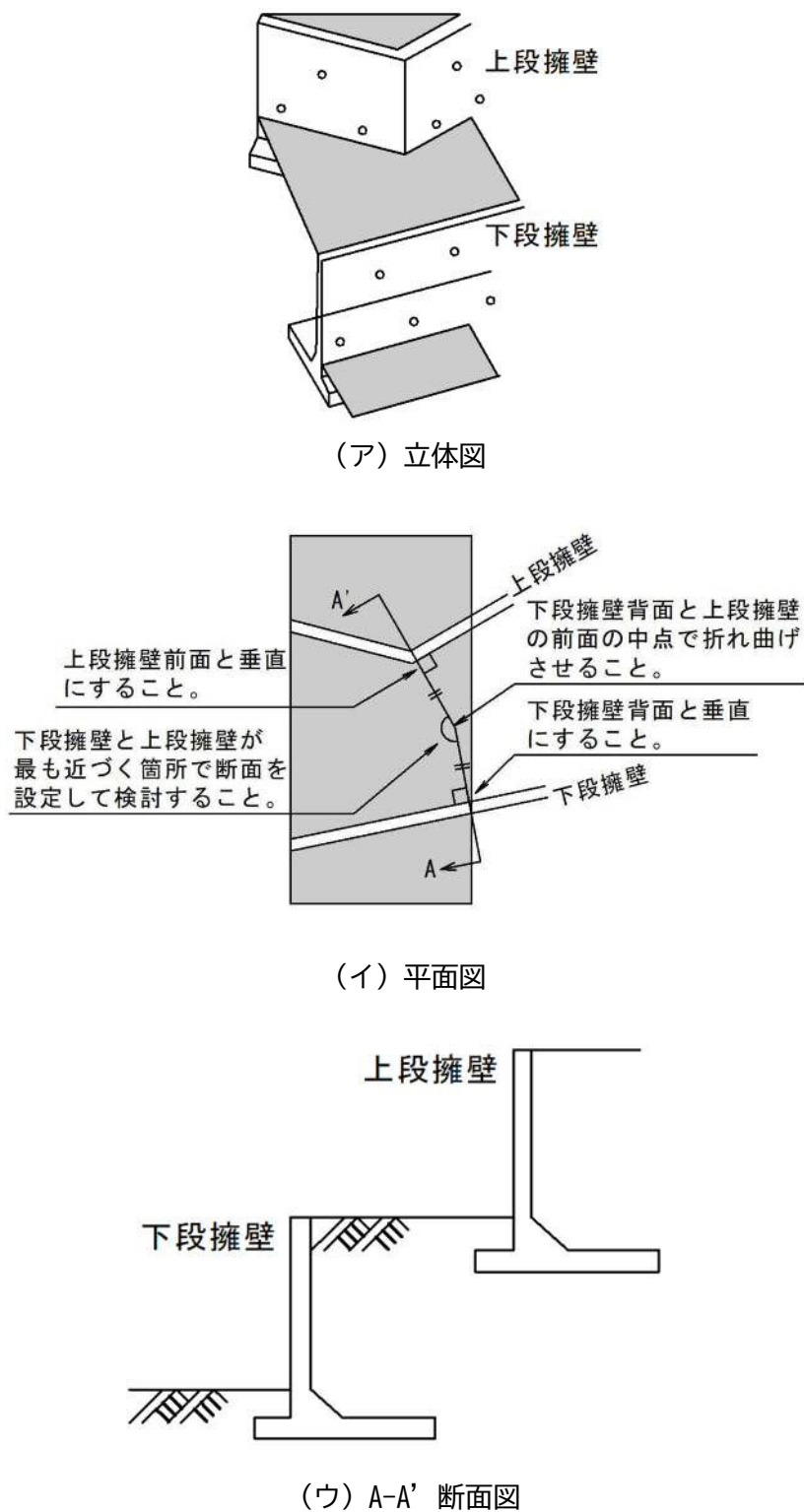
図 5-9 上下の擁壁が平行でない場合の検討断面の設定
