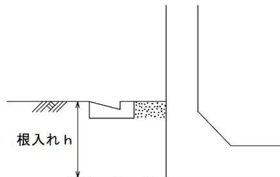
図 5-29 前面にL形側溝がある場合の根入れ
