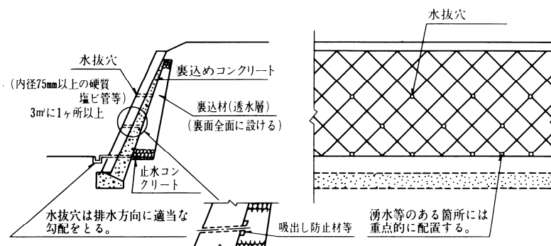
図 5-18 練積み造擁壁の水抜穴配置図
