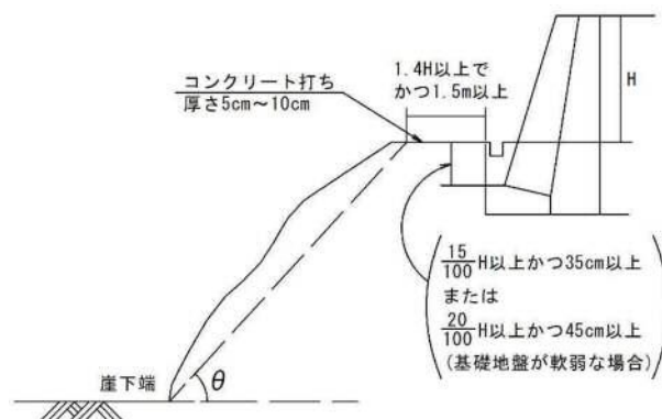
図 5-4 斜面上に擁壁を設置する場合
