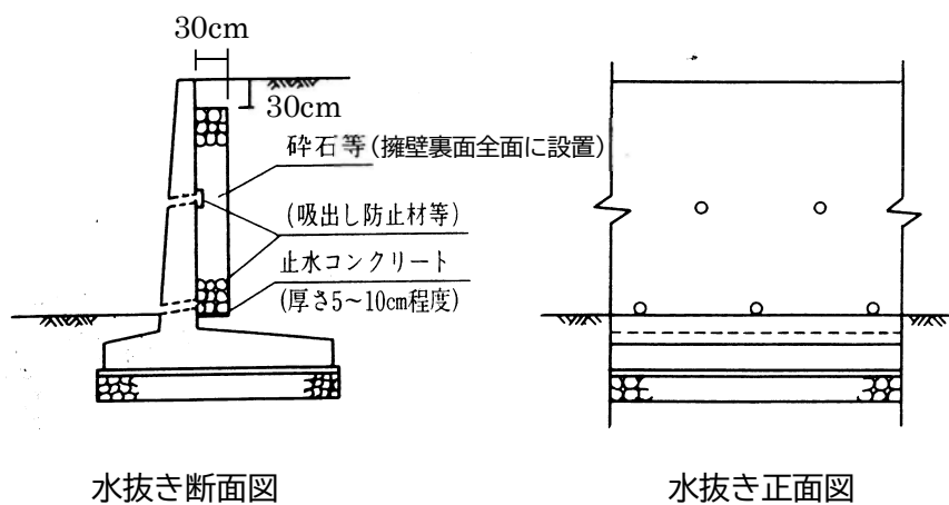
図 5-19 鉄筋コンクリート造等の水抜き穴配置図
