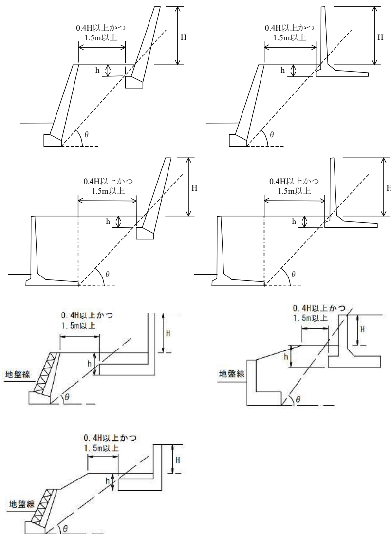
図 5-5 二段擁壁の場合（その 1）
