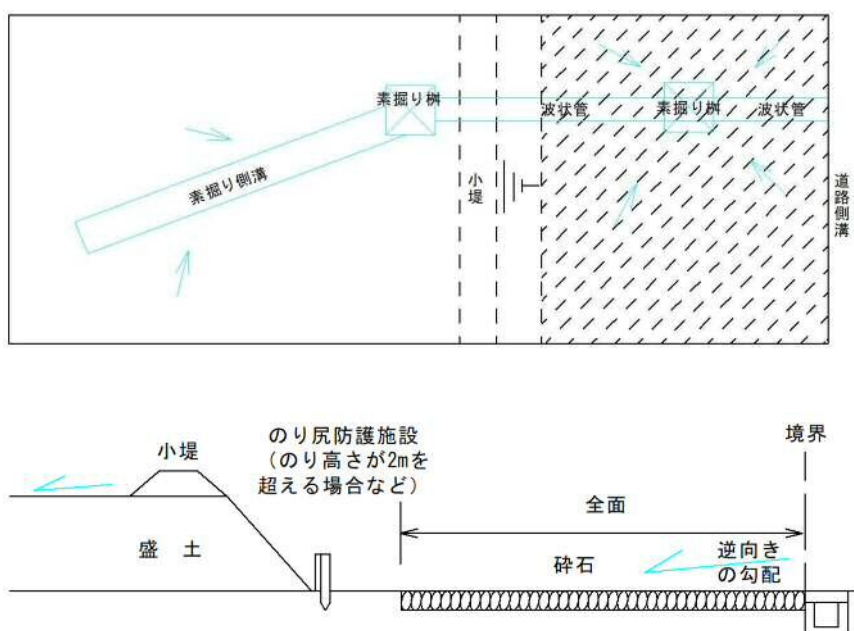
図 10-2 1 次造成時の対策例②
