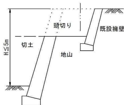
図 5-8 やむを得ず二段積み擁壁となる場合の例
