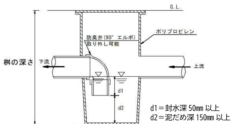
図 3-3 防臭桝の一般構造
