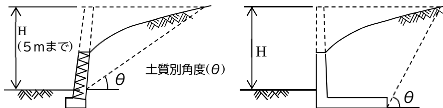
図 5-30 上部に斜面がある場合の擁壁
