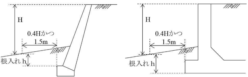
図 5-25 根入れ
