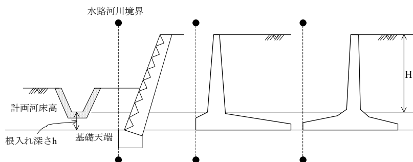
図 5-26 河川境界に隣接する場合
