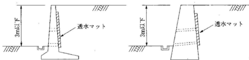
(a) 擁壁の見かけ高さが 3m 以下の場合
