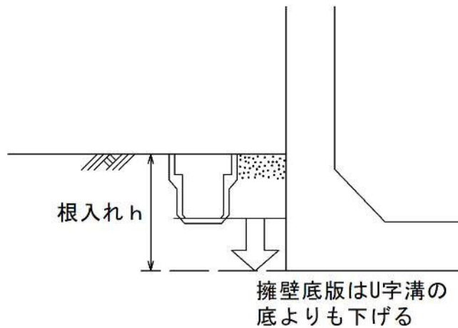
図 5-28 前面にU字溝がある場合の根入れ
