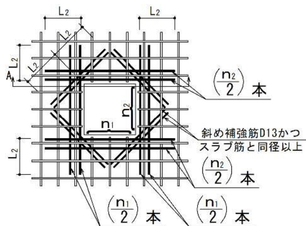
直線定着の長さ L2
