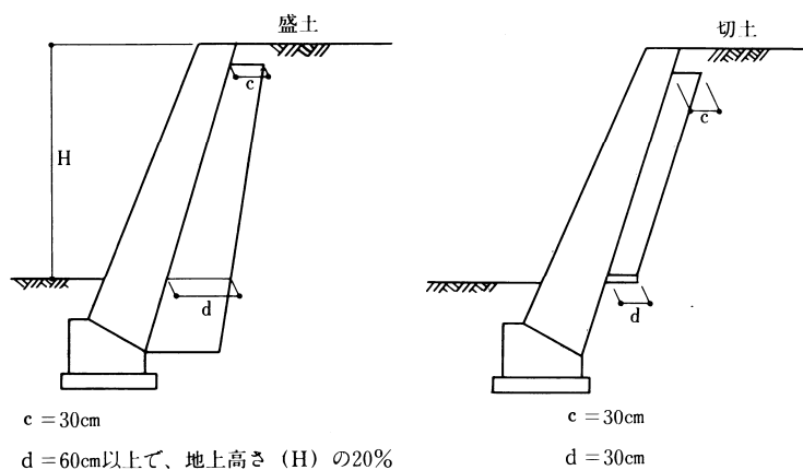
図 5-20 練積み造擁壁の裏込材
