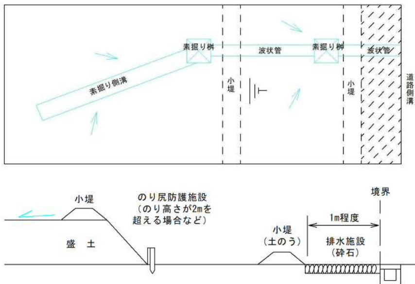
図 10-1 1 次造成時の対策例①
