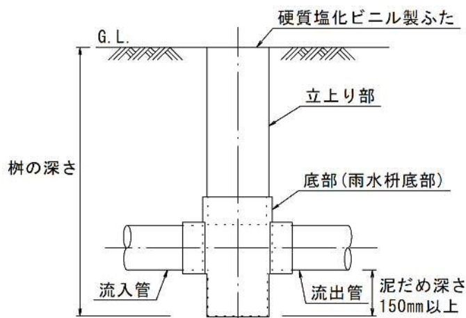
図 3-2 雨水桝の一般構造
