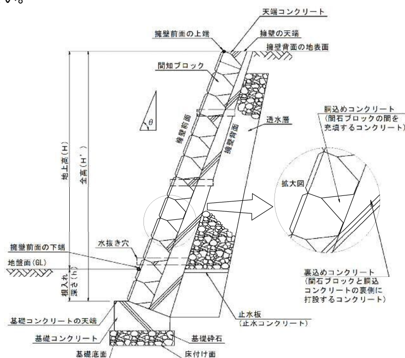
図 5-2 練積み造擁壁の構造解説図
