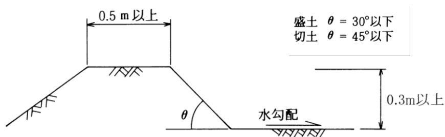
図 1-3 土えん堤（小堤）構造図
