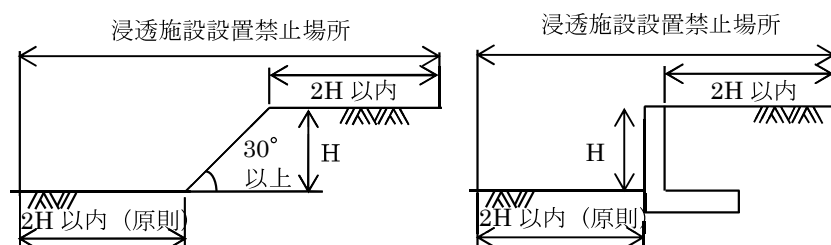
図 3-7 斜面近傍の浸透施設設置禁止場所
