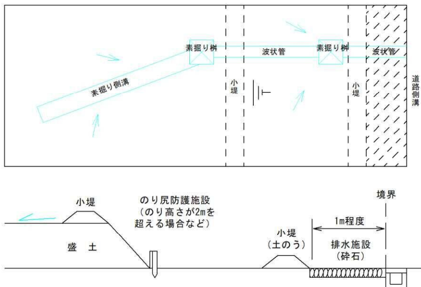
図 10-1 一次造成時の対策例①
