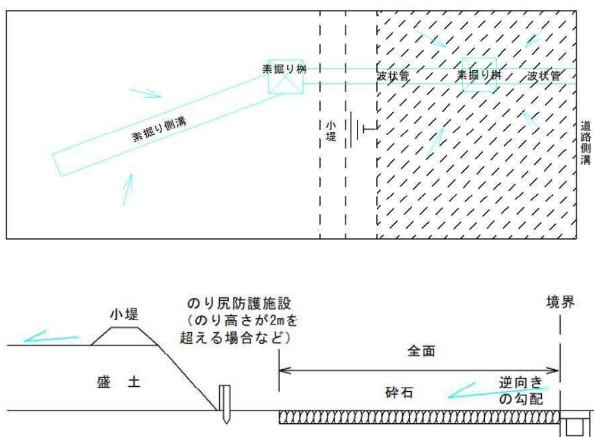
図 10-2 一次造成時の対策例②
