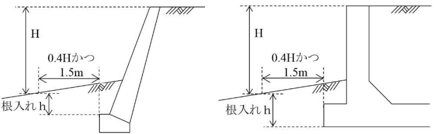
図 5-25 根入れ
