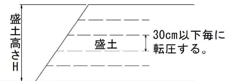
図1-4 転圧のイメージ
