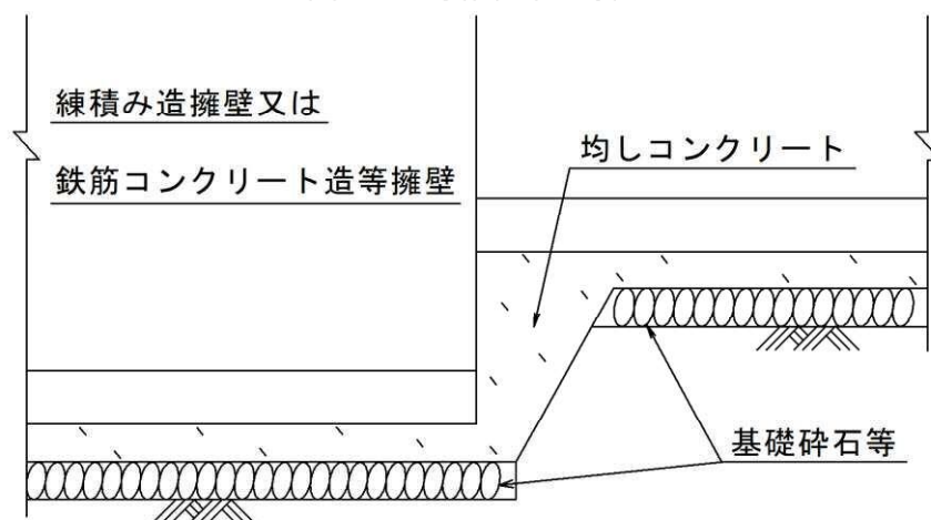
図 5-12 段切りした部分の基礎構造
