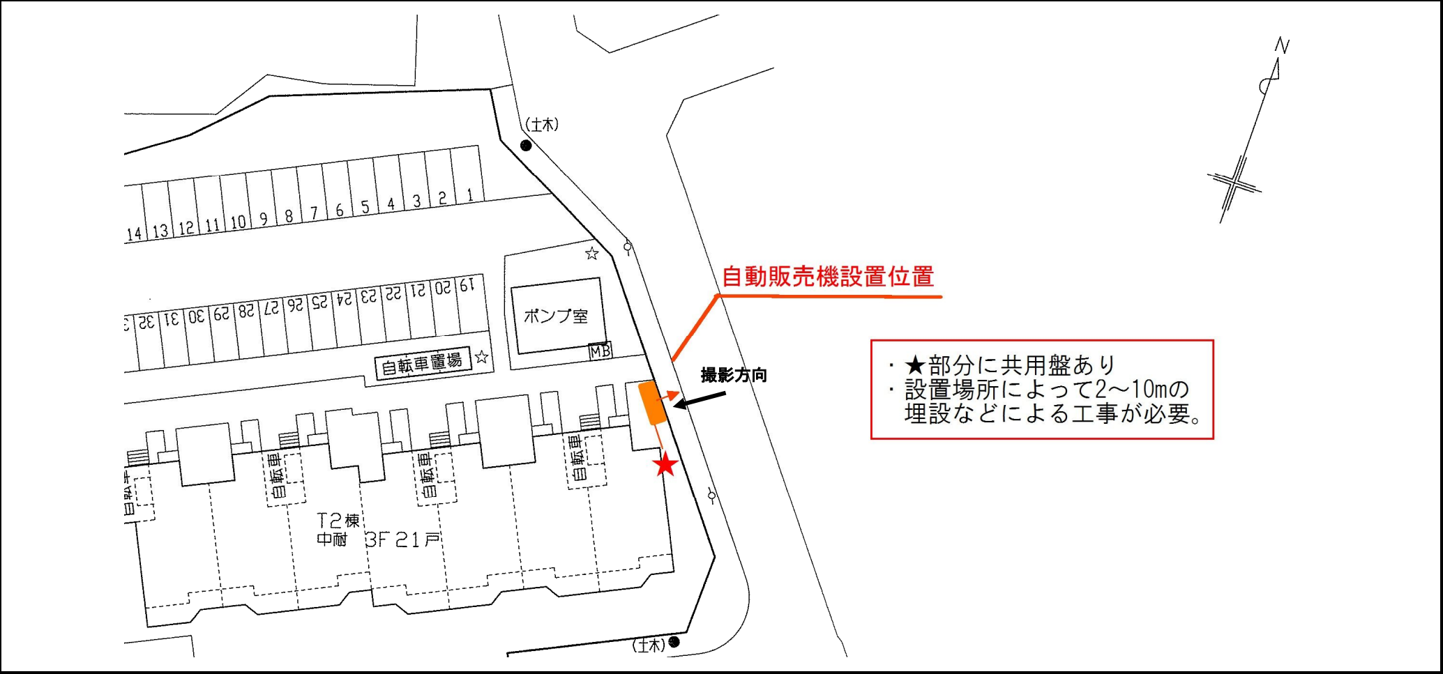
配置図及び電気工事方法
