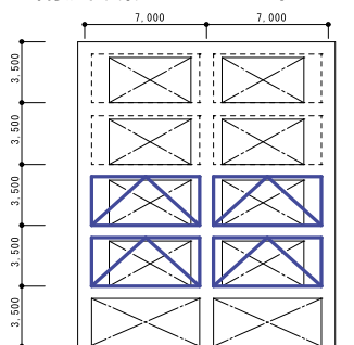
(Y1通り軸組図)
