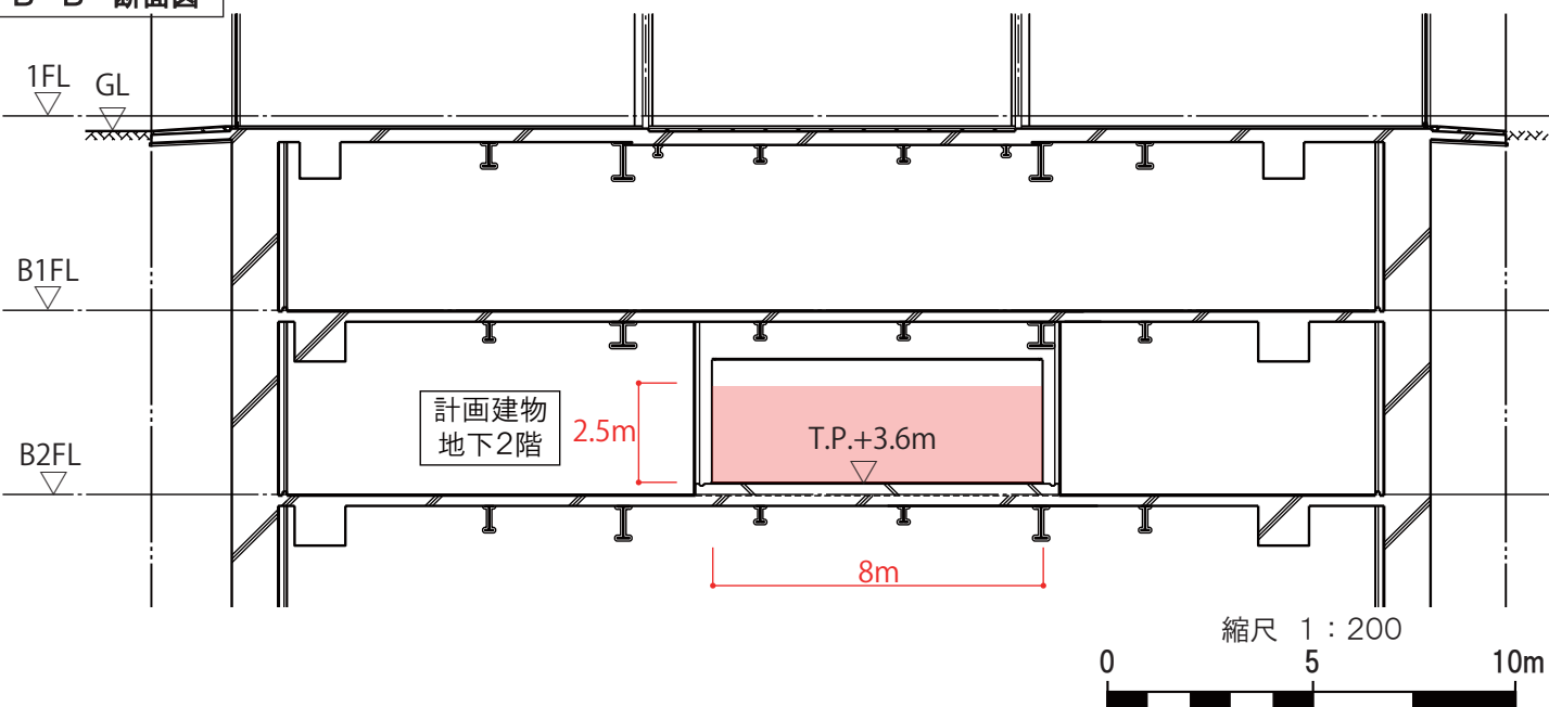
B-B' 断面図
