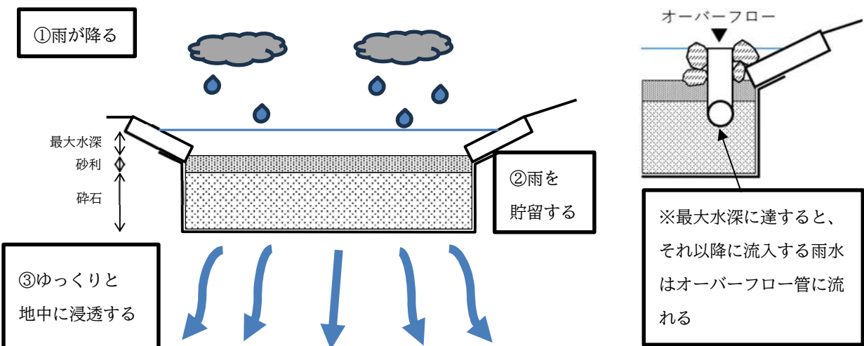
啓発スポットの雨庭の構造図と仕組み
