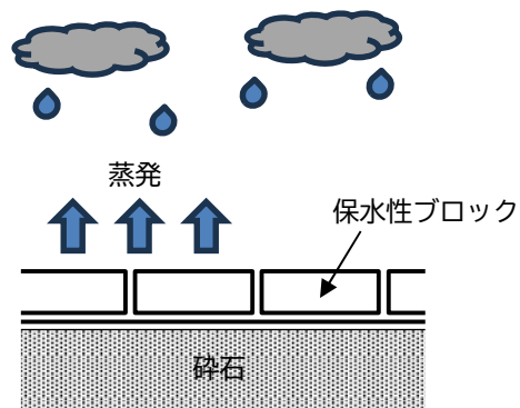
啓発スポットの保水性舗装の構造図
